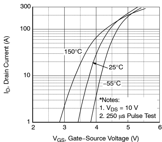
图 2. 传输特性
