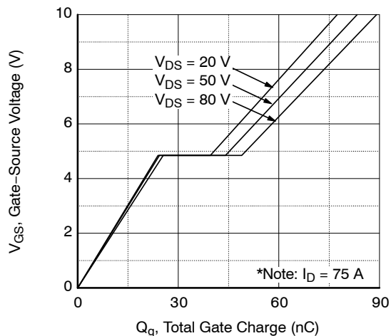
图 6. 栅极电荷
