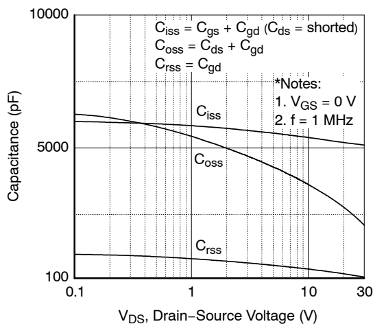
图 5. 电容特性
