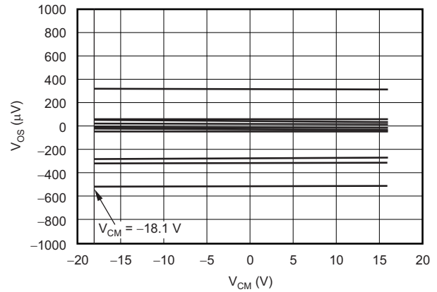
图 2. 失调电压与共模电压间的关系
