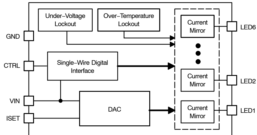
图 4. 框图
