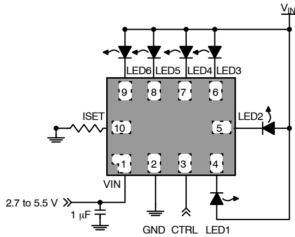
图 3. FAN5626 6 LED 的典型应用
