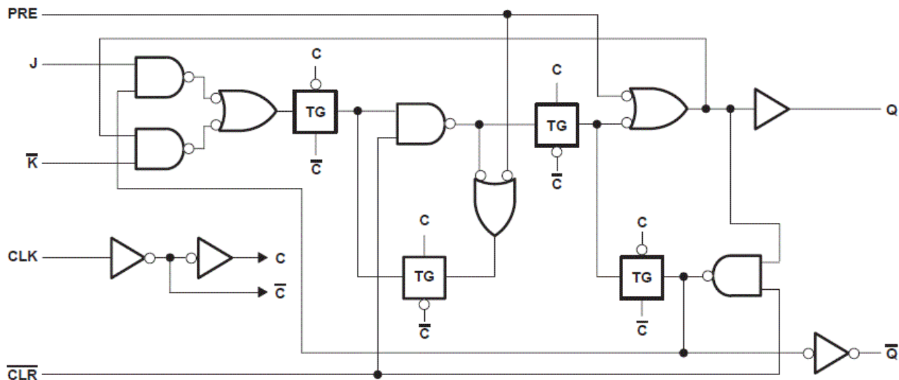
功能方框图
