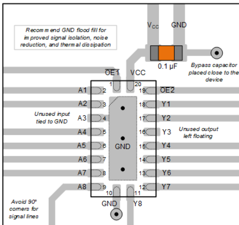
图 9-1. Layout Diagram
