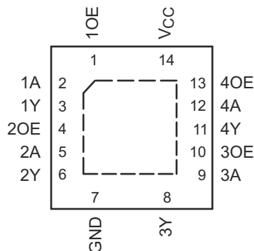
图 3-2. SN74LVC126A-Q1 BQA 封装；14 引脚 WQFN （顶视图）
