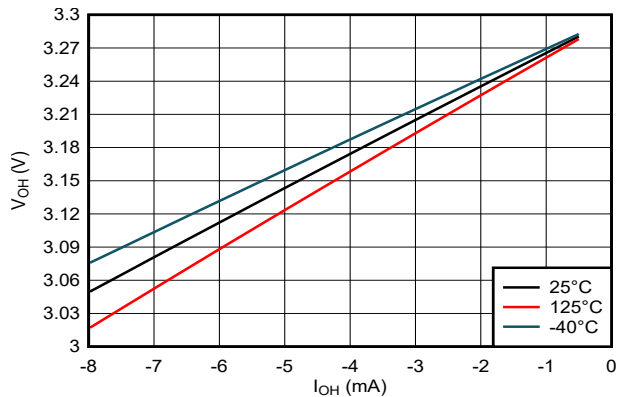
图 6-3. 高电平状态下输出电压与电流间的关系；3.3V 电源
