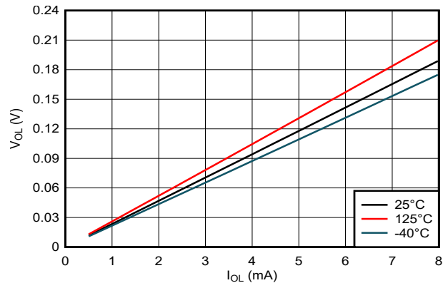
图 6-4. 低电平状态下输出电压与电流间的关系；3.3V 电源
