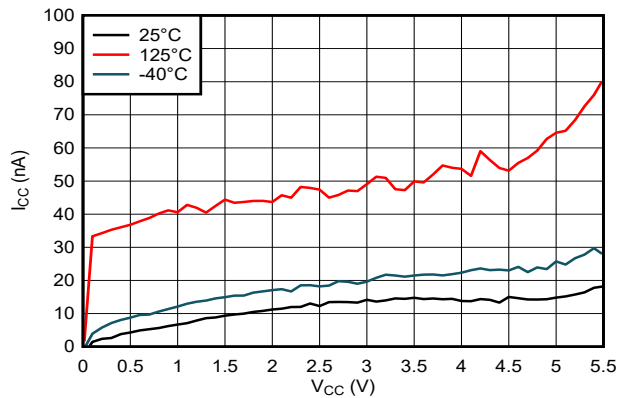
图 6-1. 电源电流与电压电源的电压间的关系
