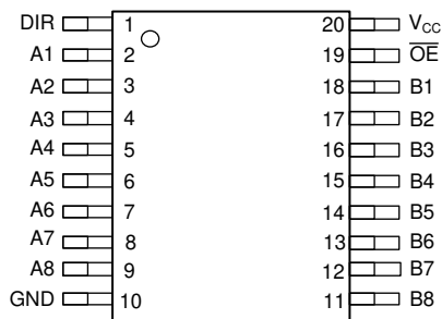
图 5-1. SN74AHC245-Q1 PW 封装，20 引脚 TSSOP (顶视图)
