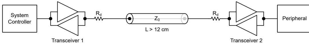
图 9-1. 应用方框图
