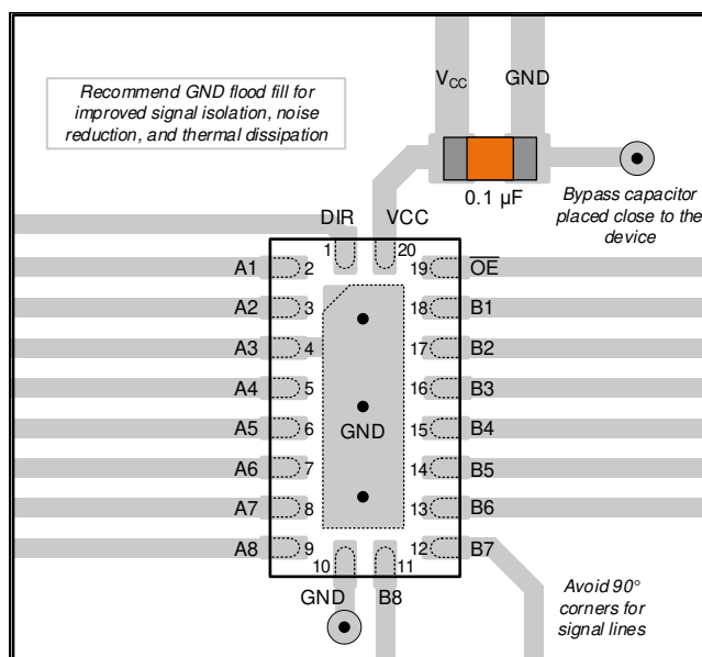
图 9-3. 采用 RKS 封装的 SN74AHC245-Q1 的示例布局
