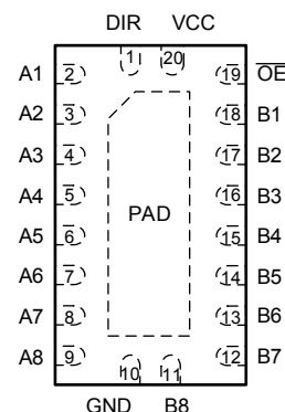
图 5-2. SN74AHC245-Q1 WRKS 封装，20 引脚 WQFN (顶视图)
