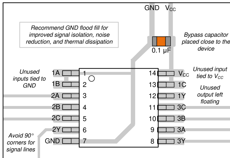
图 7-1. SN74LV11A 的示例布局
