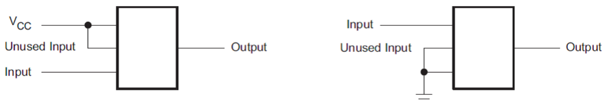
图 7-1. Layout Example
