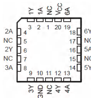
图 5-2. SN54ACT04 FK Package Top View
