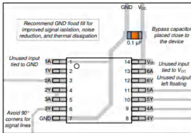
图 9-1. Layout Diagram
