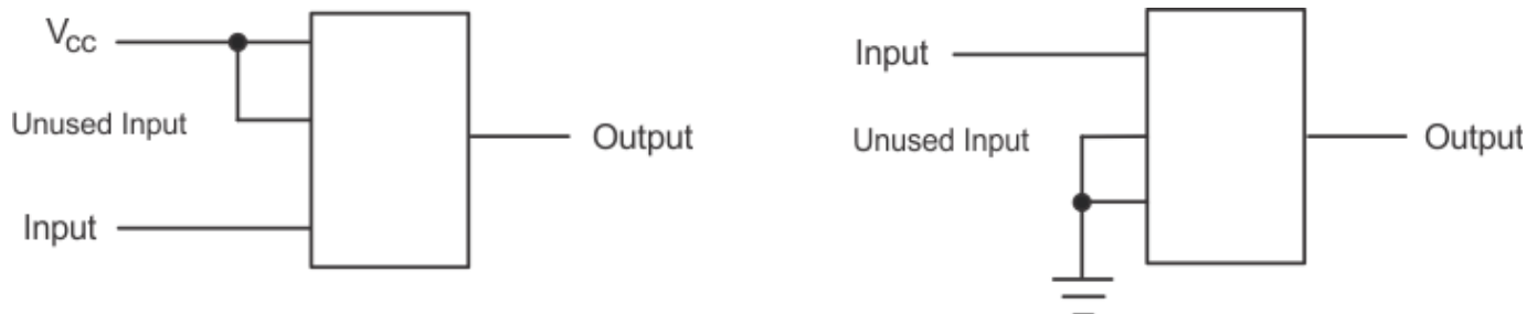
图 9-3. Layout Diagram
