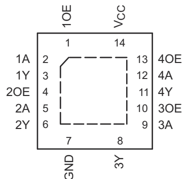
图 4-2. SN74LVC126A BQA 或 RGY 封装；14 引脚 WQFN 或 VQFN (顶视图)
