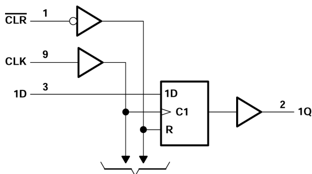
图 3-1. 逻辑图 (正逻辑)
