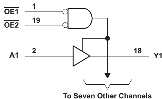
功能方框图
