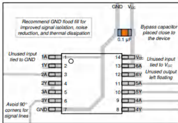
图 9-1. Layout Diagram
