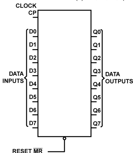
功能方框图
