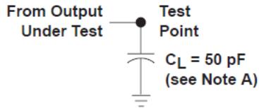
图 7-1. Load Circuit
