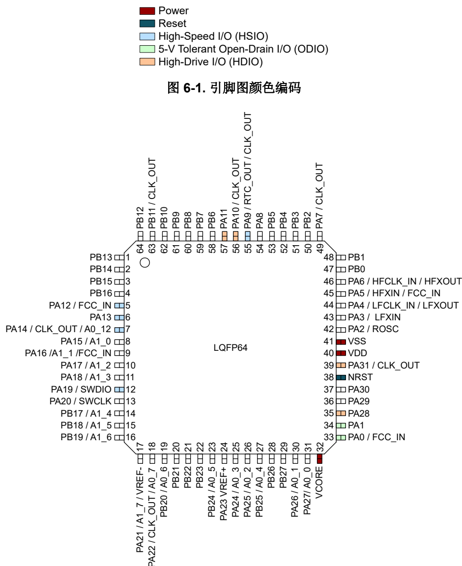
图 6-2. 64 引脚 PM (LQFP) (顶视图)
