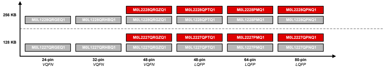
图 5-1. 器件比较图
