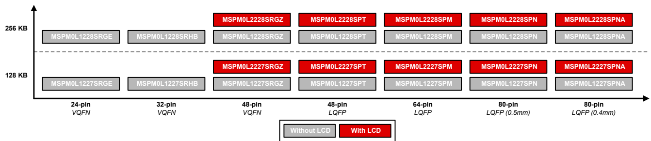
图 5-1. 器件比较图
