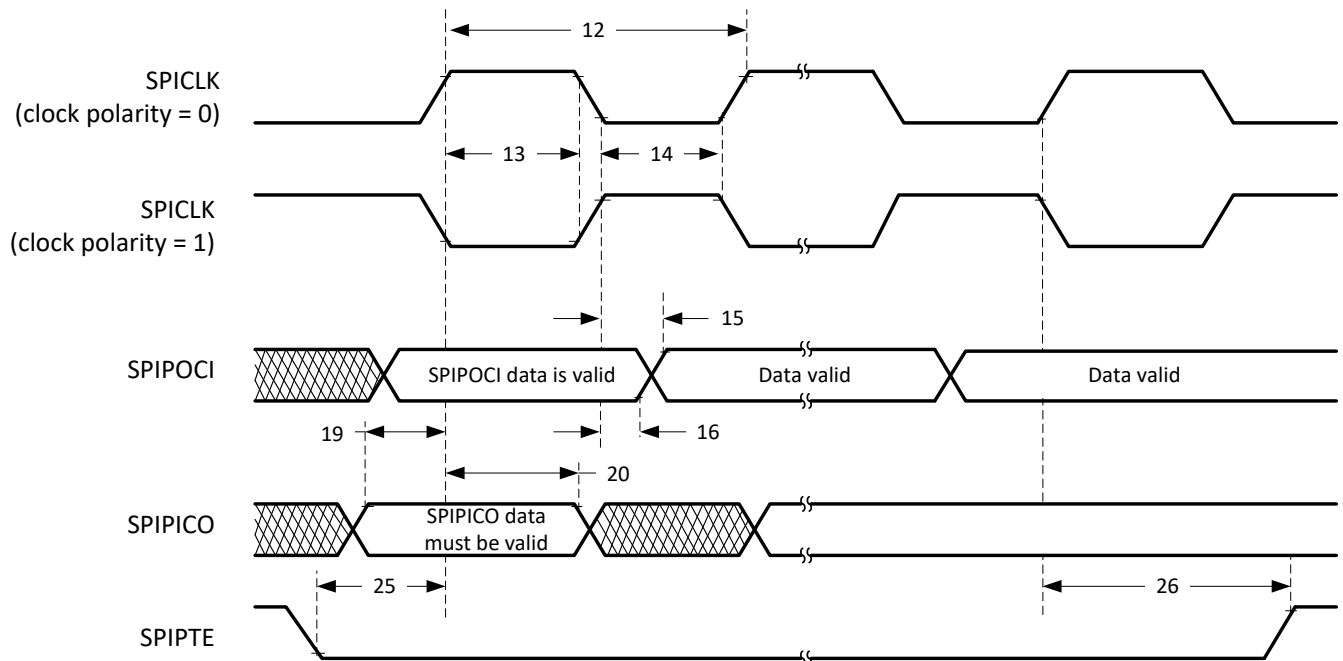
图 6-67. SPI 外设模式外部时序 ( 时钟相位 = 1 )
