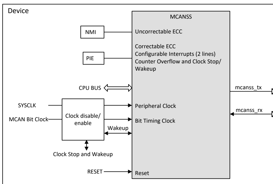
图 6-58. MCAN 模块概述
