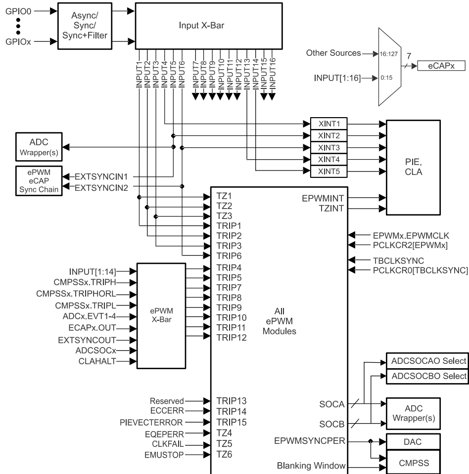
图 6-51. ePWM 跳变输入连接
