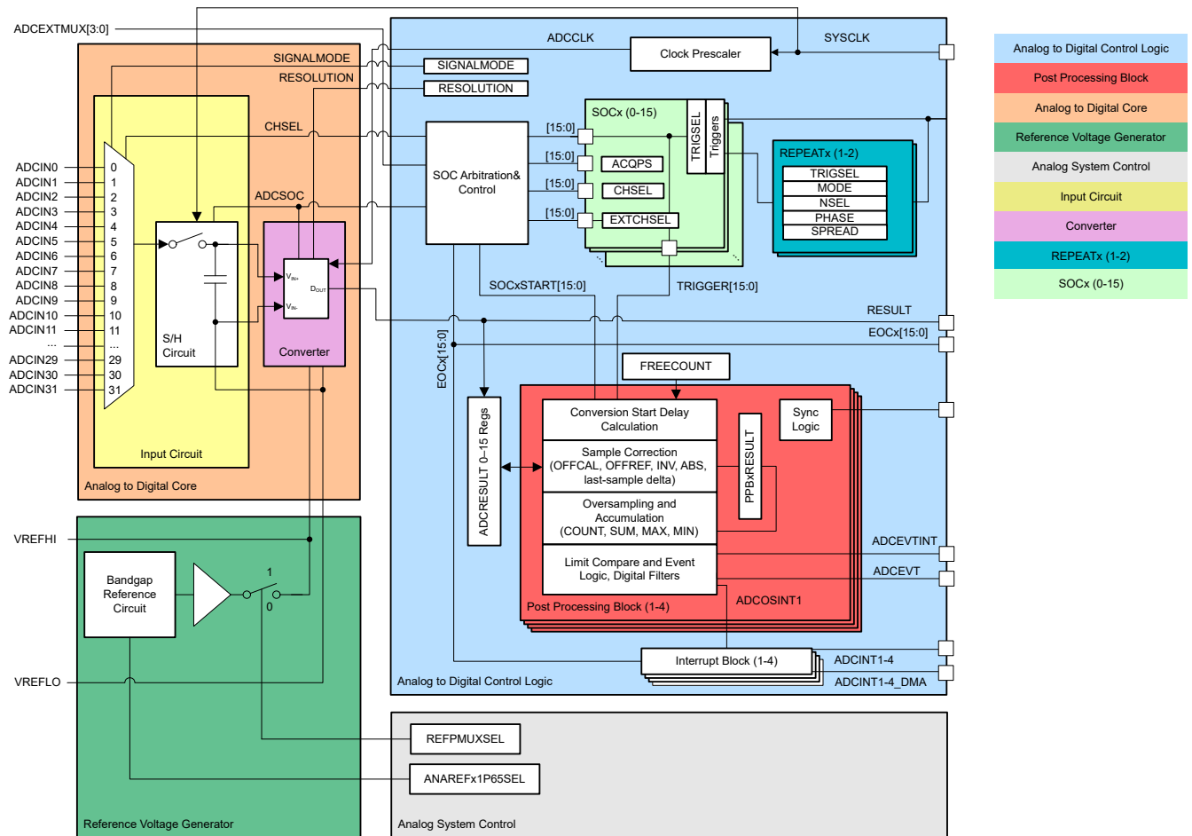
图 6-34. ADC 模块方框图
