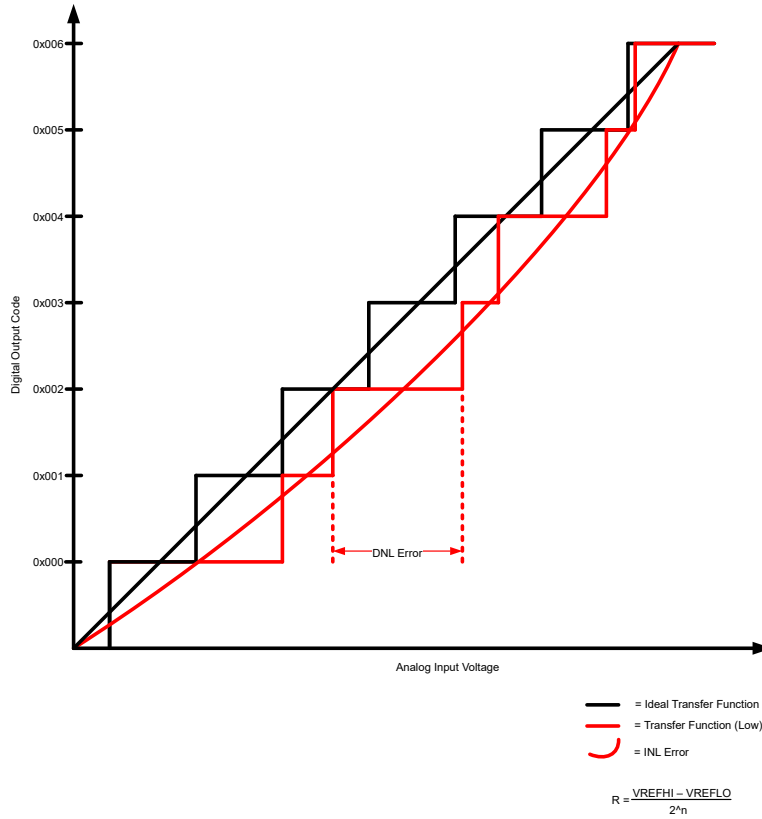
图 6-36. ADC INL 和 DNL
