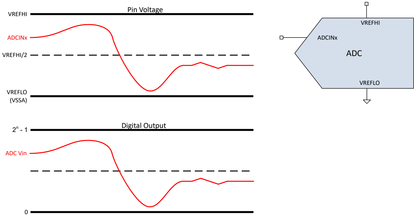
图 6-35. 单端信号模式
