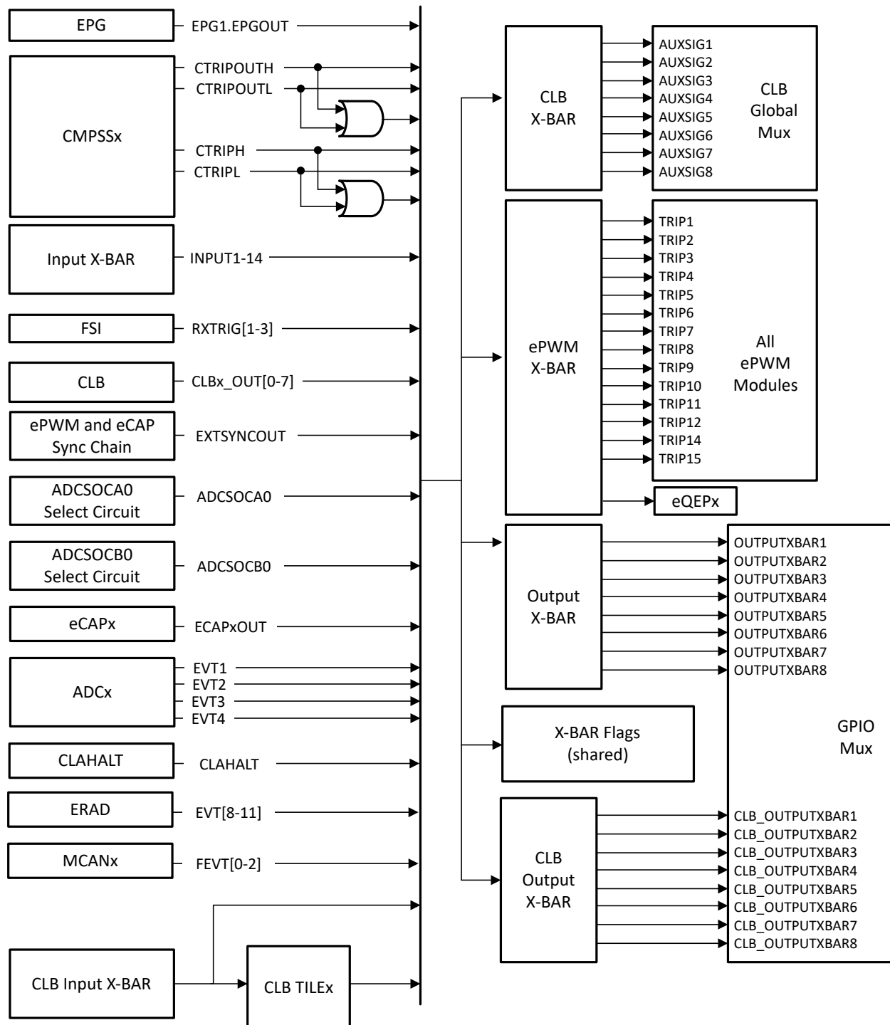
图 5-7. 输出 X-BAR、CLB X-BAR、CLB 输出 X-BAR 和 ePWM X-BAR 源
