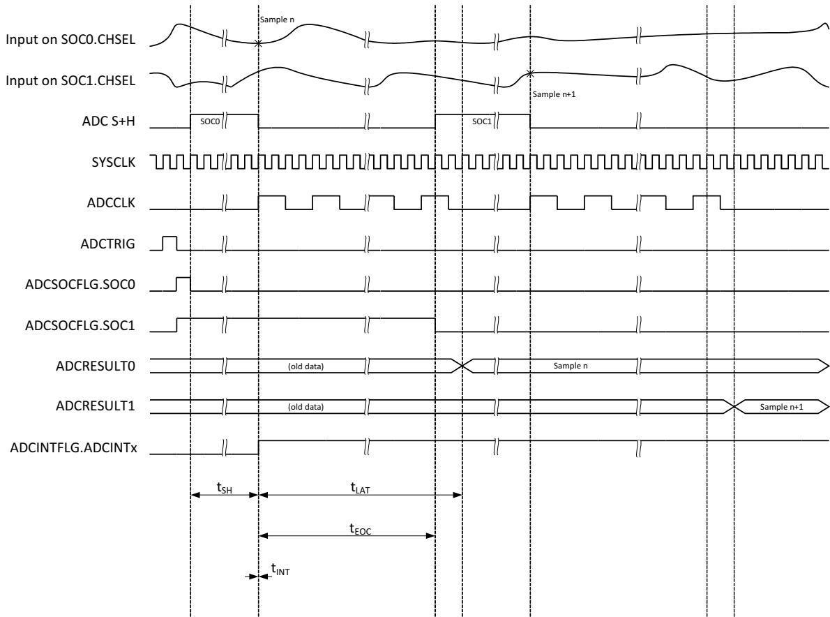
图 6-38. 提前中断模式下 12 位模式的 ADC 时序
