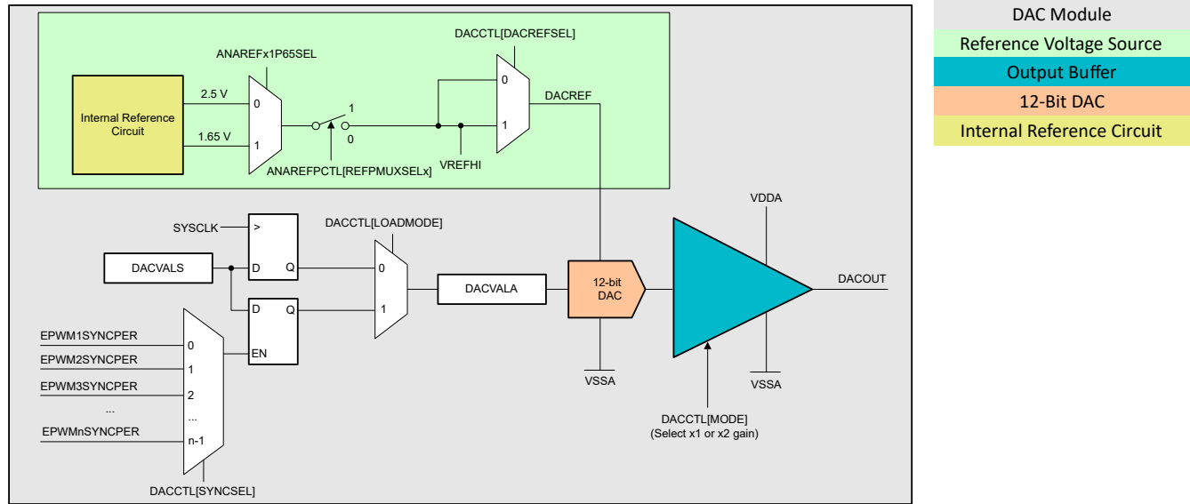
图 6-48. DAC 模块方框图
