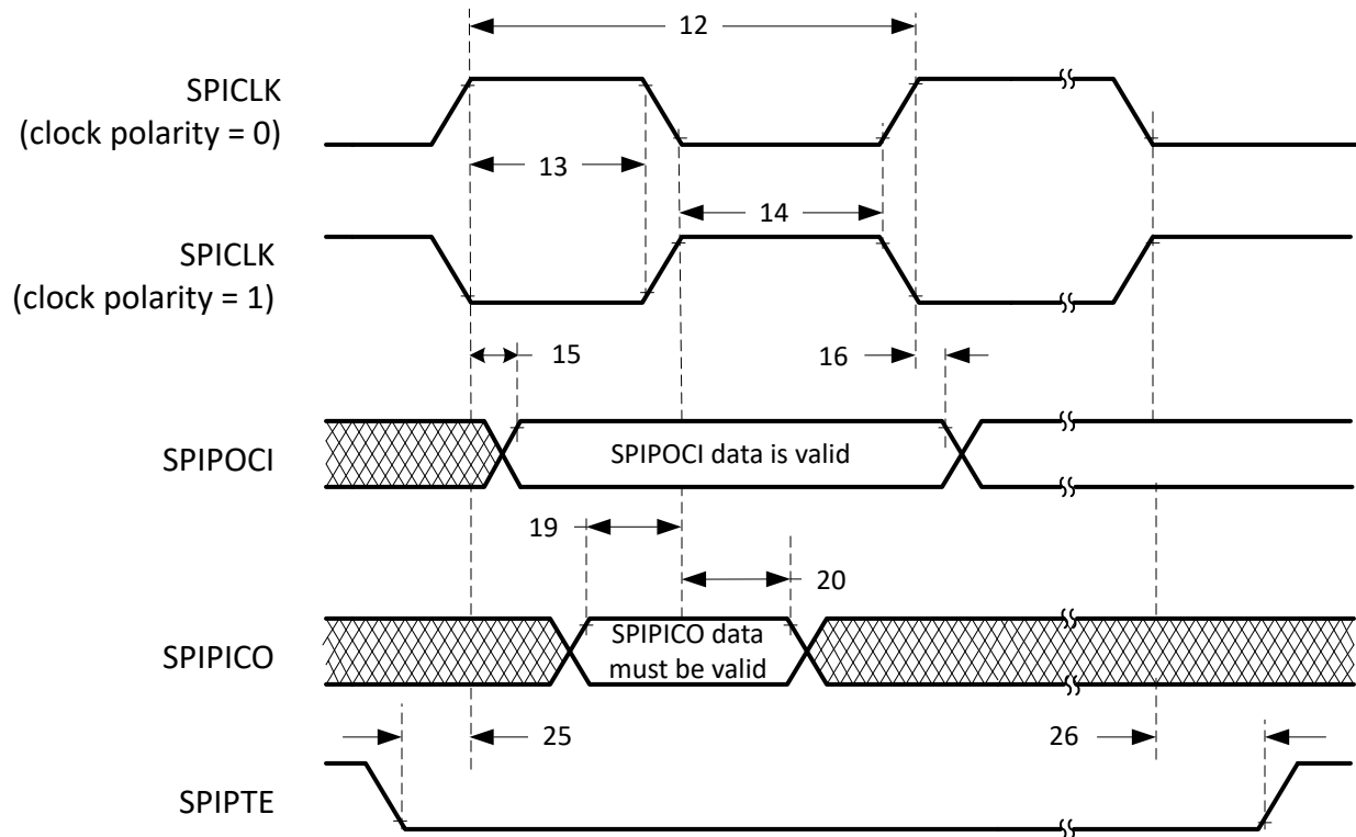
图 6-66. SPI 外设模式外部时序 ( 时钟相位 = 0 )
