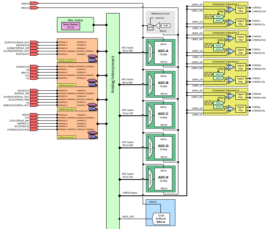
图 6-32. 模拟子系统方框图 ( 100 引脚封装 )
