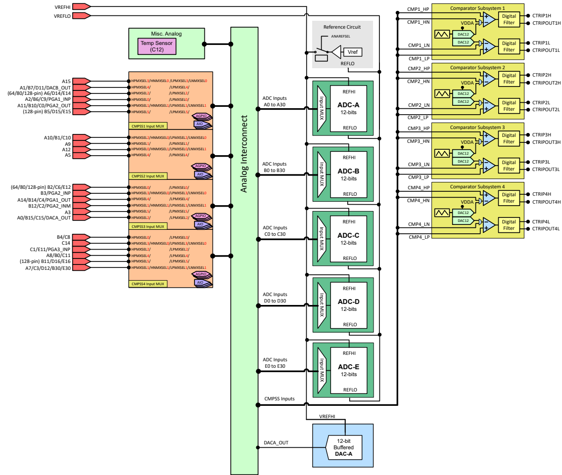
图 6-31. 模拟子系统方框图 ( 128/80/64/56 引脚封装 )
