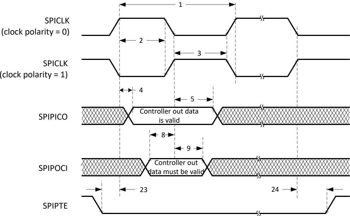
图 6-64. SPI 控制器模式外部时序 (时钟相位 = 0)
