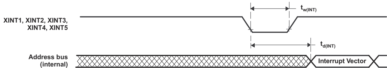
图 6-27. 外部中断时序
