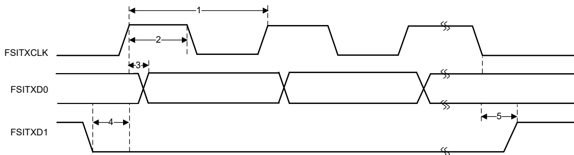
图 6-75. FSITX SPI 信令模式时序
