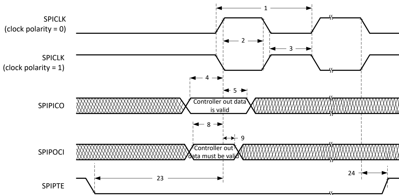
图 6-65. SPI 控制器模式外部时序 ( 时钟相位 = 1 )
