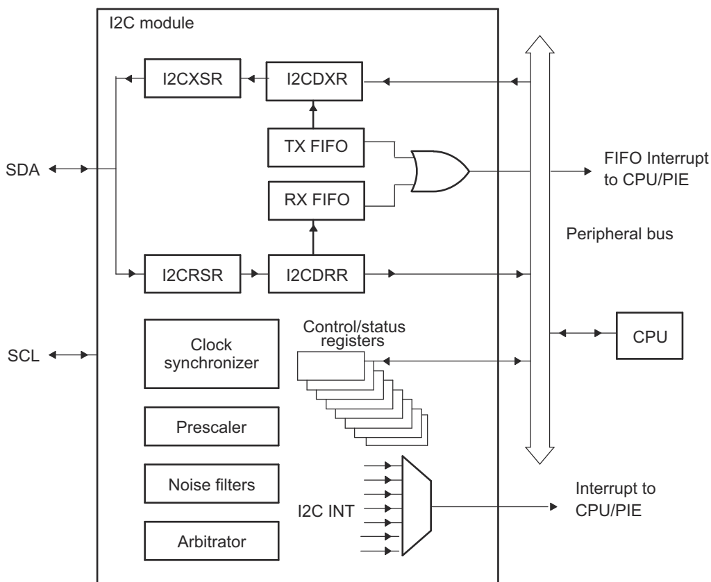
图 6-59. I2C 外设模块接口
