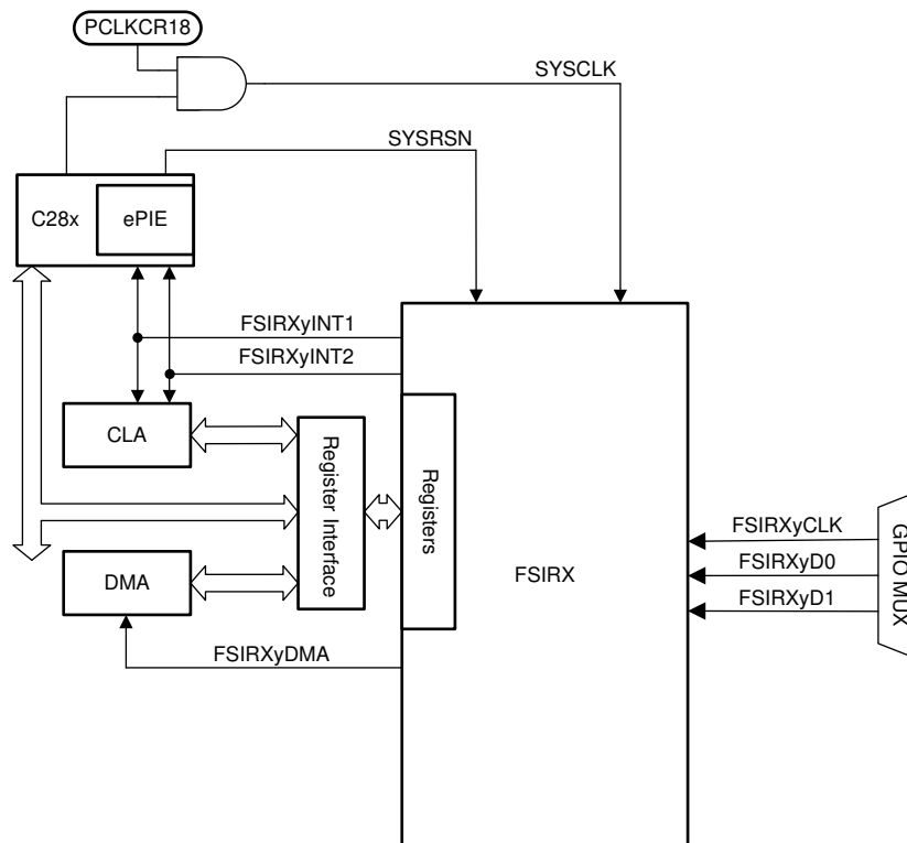
图 6-72. FSIRX CPU 接口
