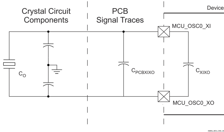
图 6-19. 并联电容
