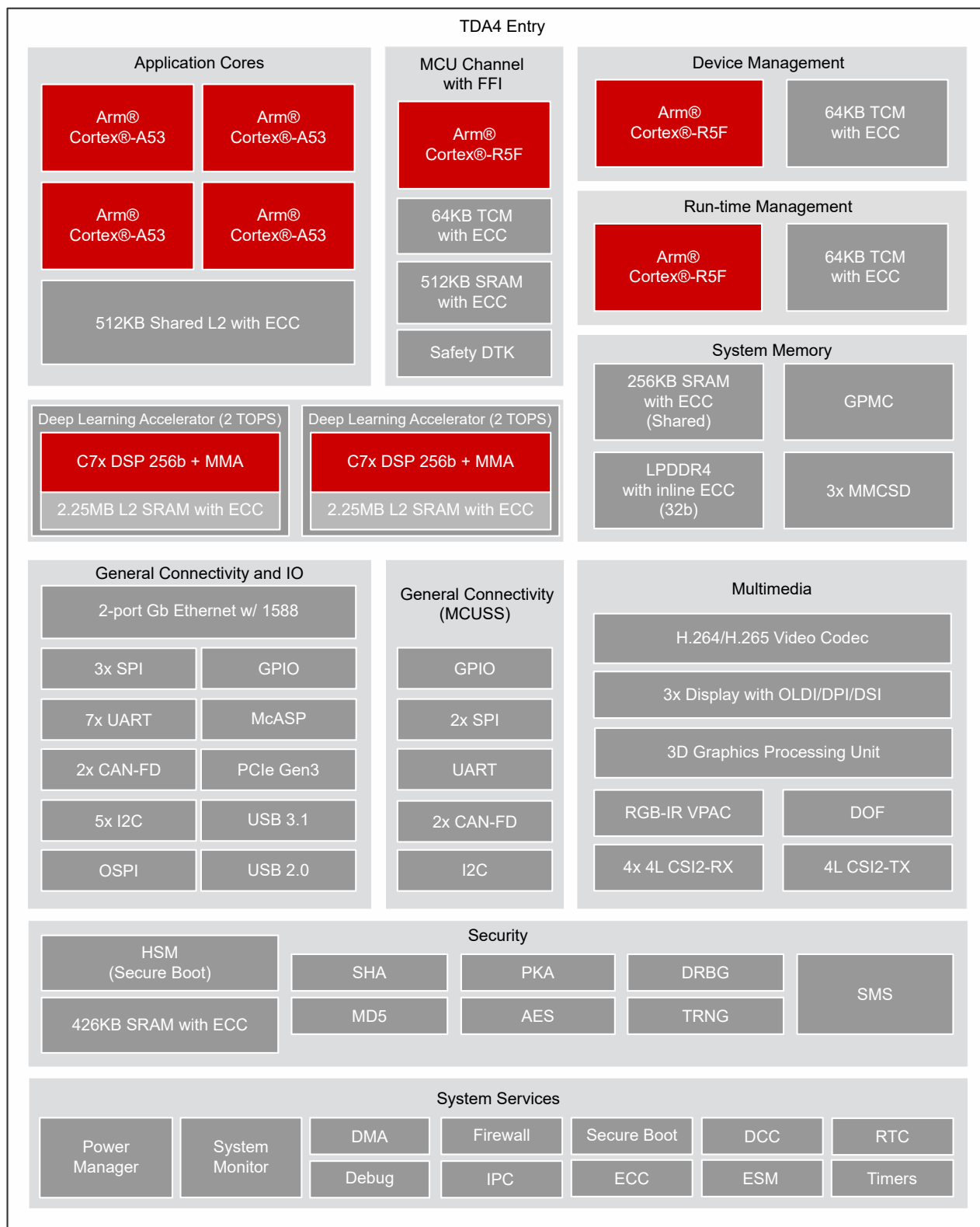
图 3-1. 功能方框图
