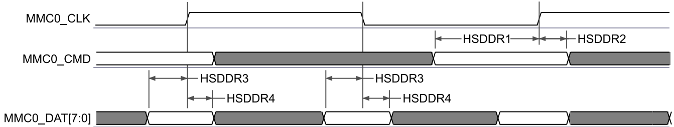
图 6-72. MMC0 - 高速 DDR 模式 - 接收模式
