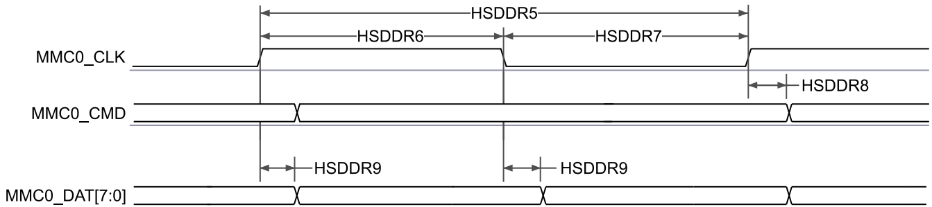
图 6-73. MMC0 - 高速 DDR 模式 - 发送模式
