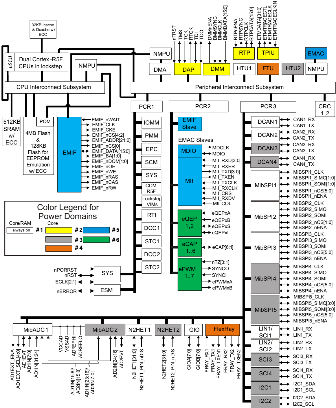
图 3-1. 功能方框图
