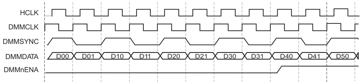
图 7-37. DMMnENA Timing
