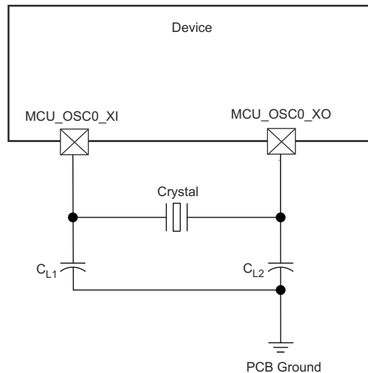
图 7-16. MCU_OSC0 Crystal Implementation
