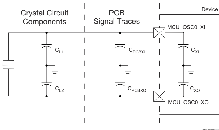
图 7-18. Load Capacitance
