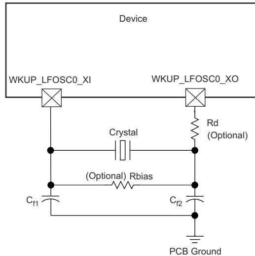
图 7-21. WKUP_LFOSC0 Crystal Implementation
