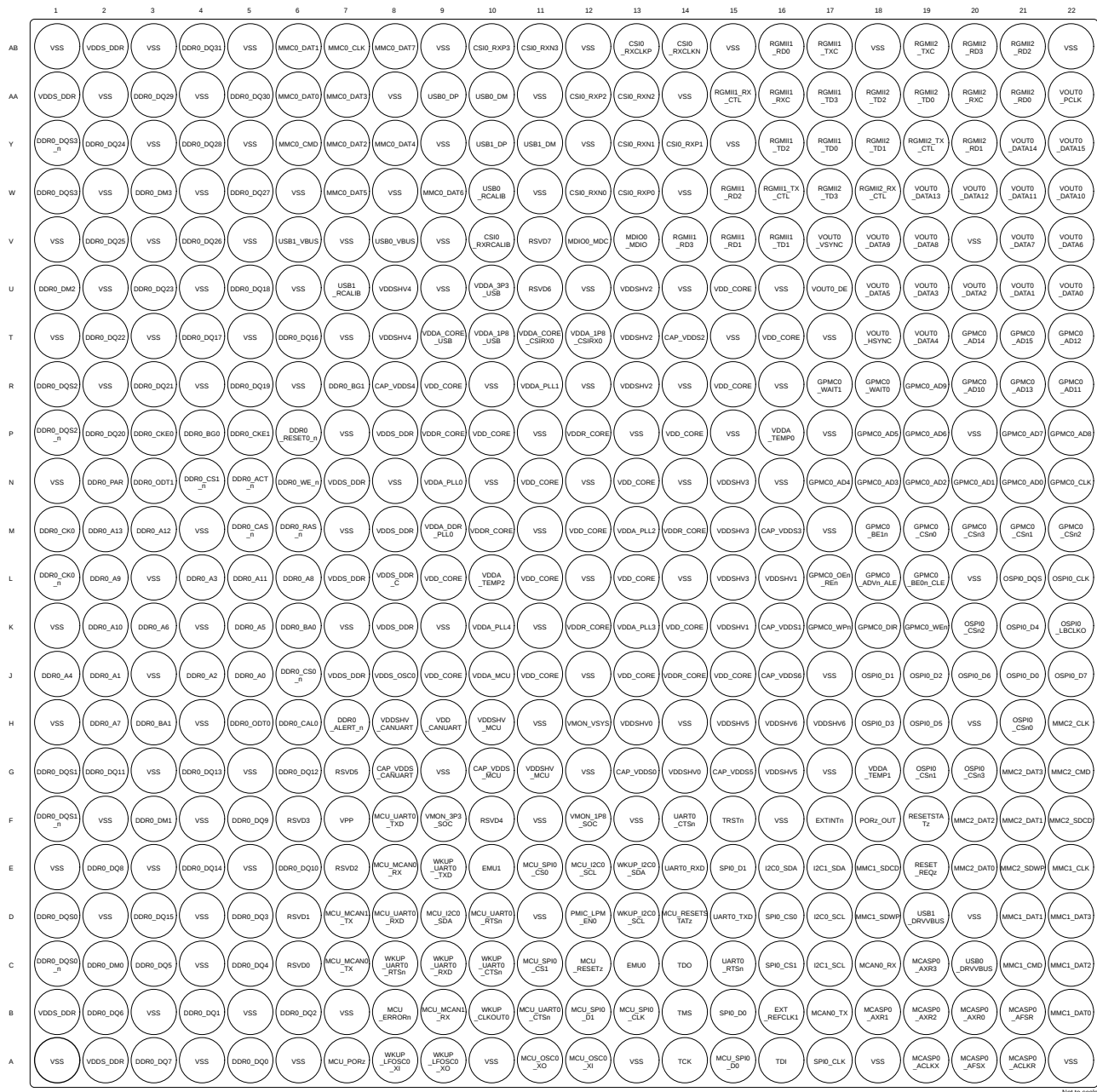
图 6-1. AMB FCBGA-N484 Pin Diagram (Bottom View)
