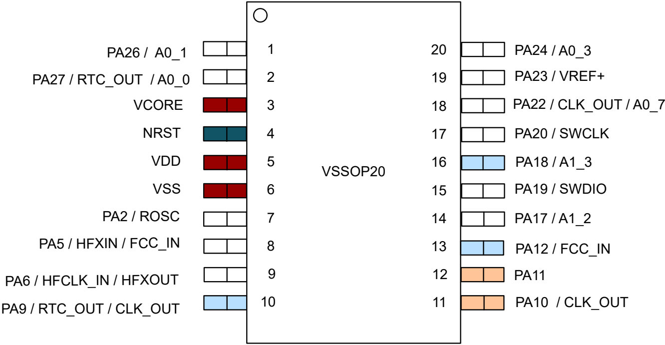
图 6-4. 20 引脚 DGS20 (VSSOP) ( 顶视图 )
