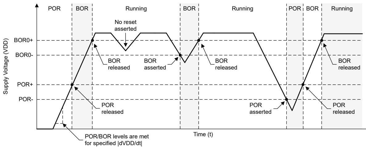
图 7-1. 下电上电 POR/BOR 条件
