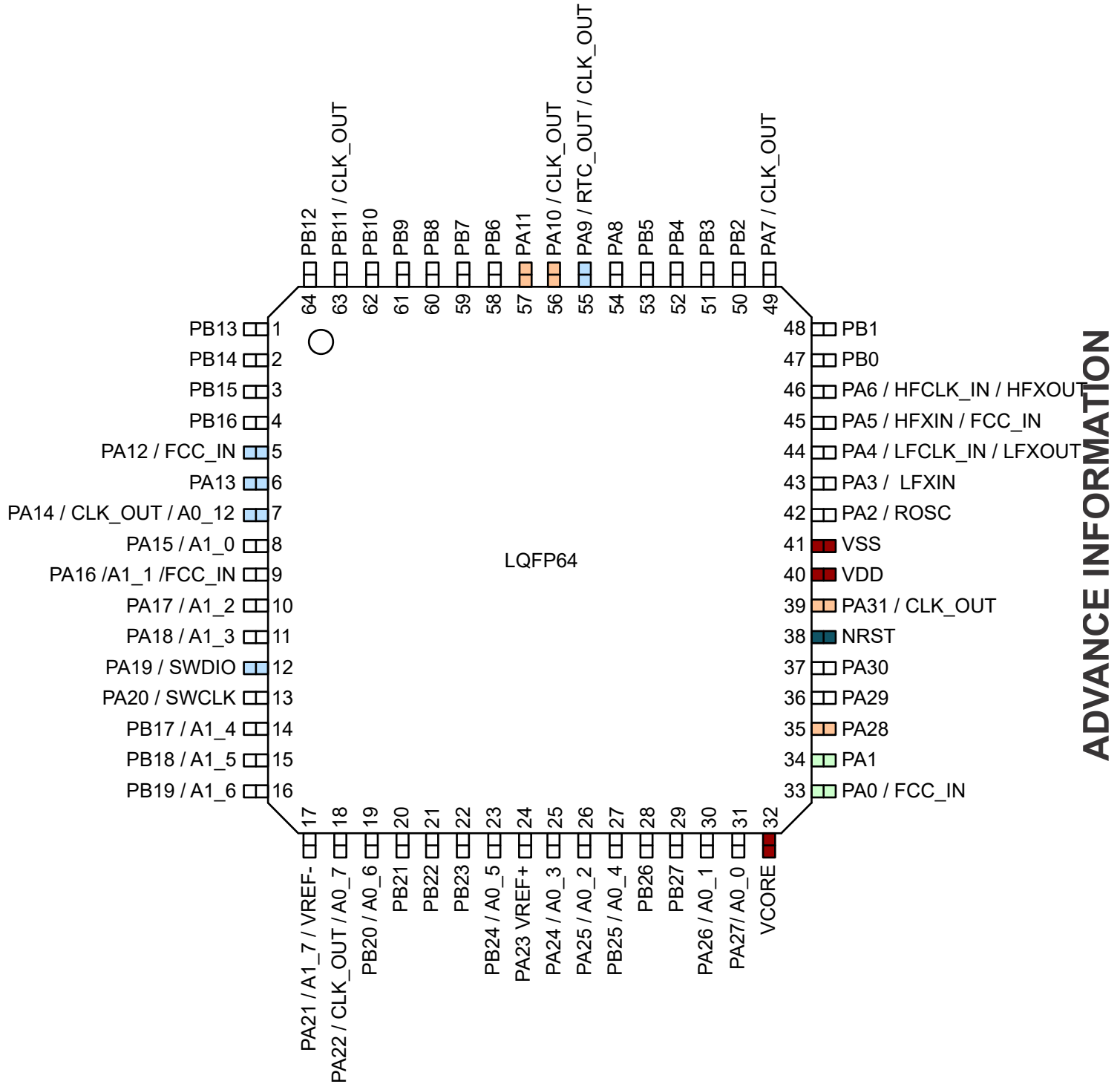
图 6-2. 64 引脚 PM (LQFP) (顶视图)
