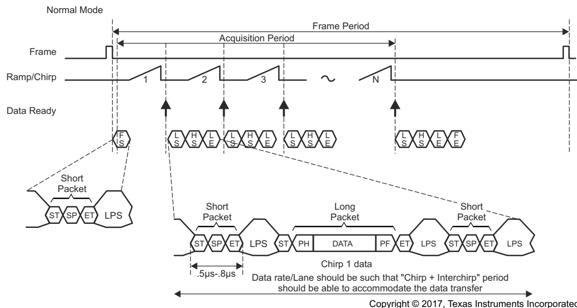
图 7-1. CSI-2 Transmission Format
