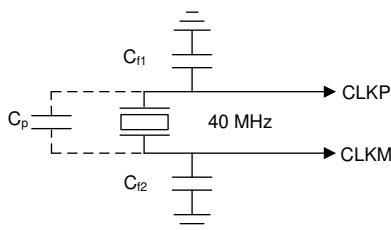
图 6-2. Crystal Implementation
