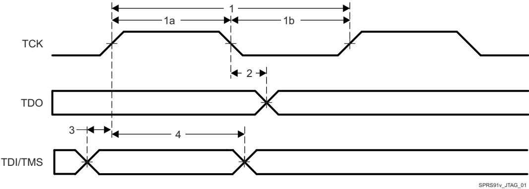
图 6-23. JTAG Timing
