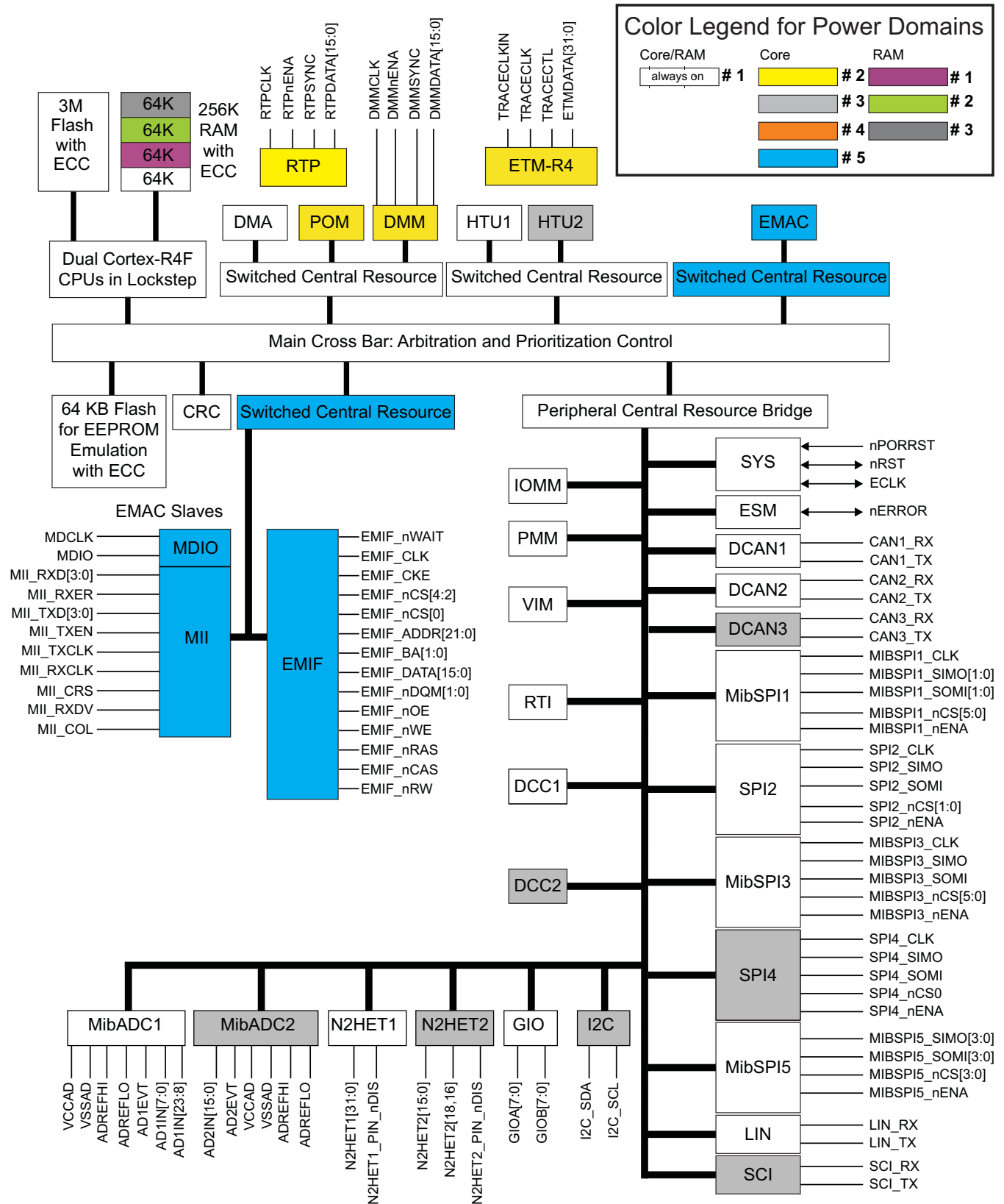
图 1-1. 功能方框图
