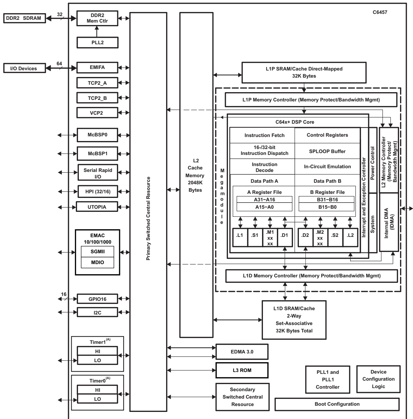
图 1-1. 功能框图
