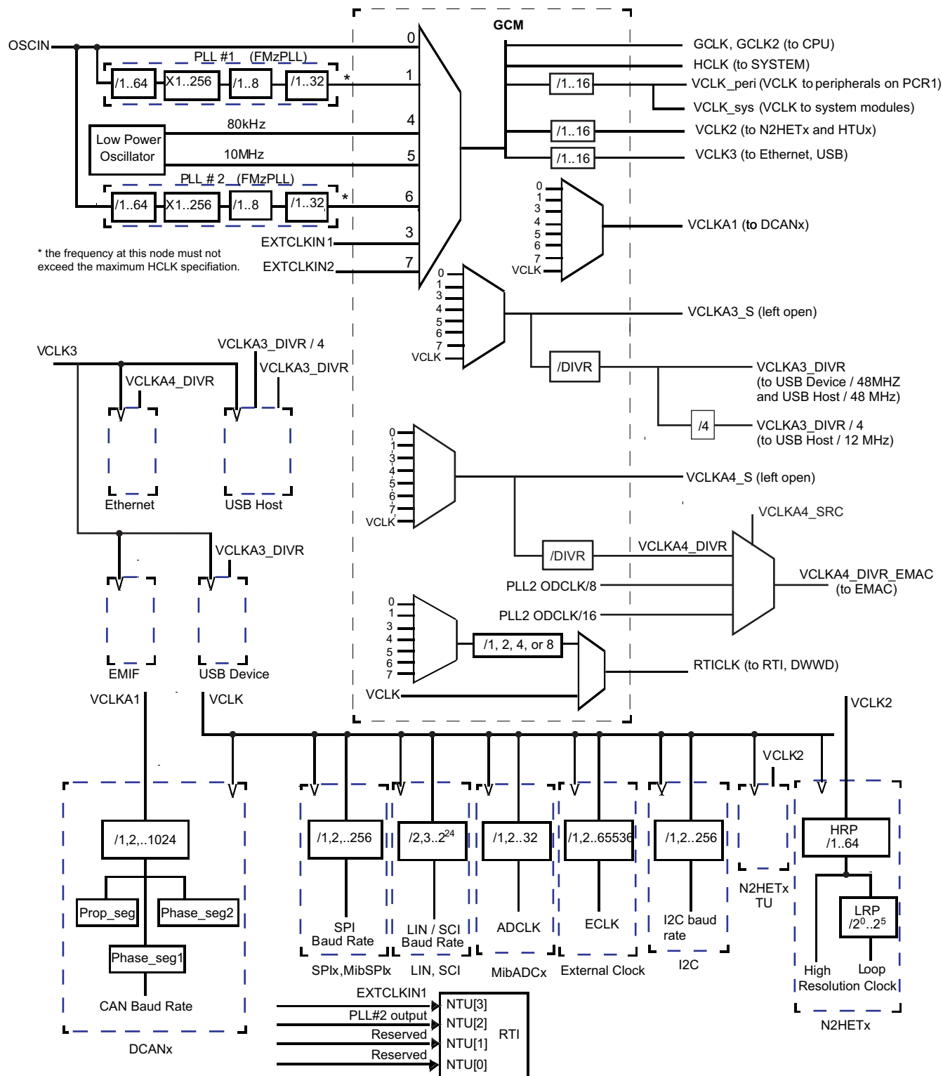
图 5-7. 器件时钟域
