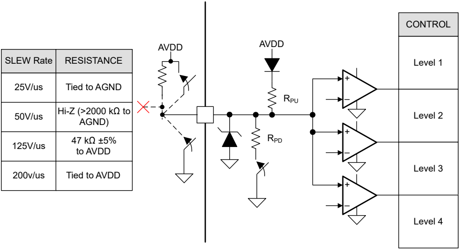
图 6-3. SLEW 输入引脚结构
