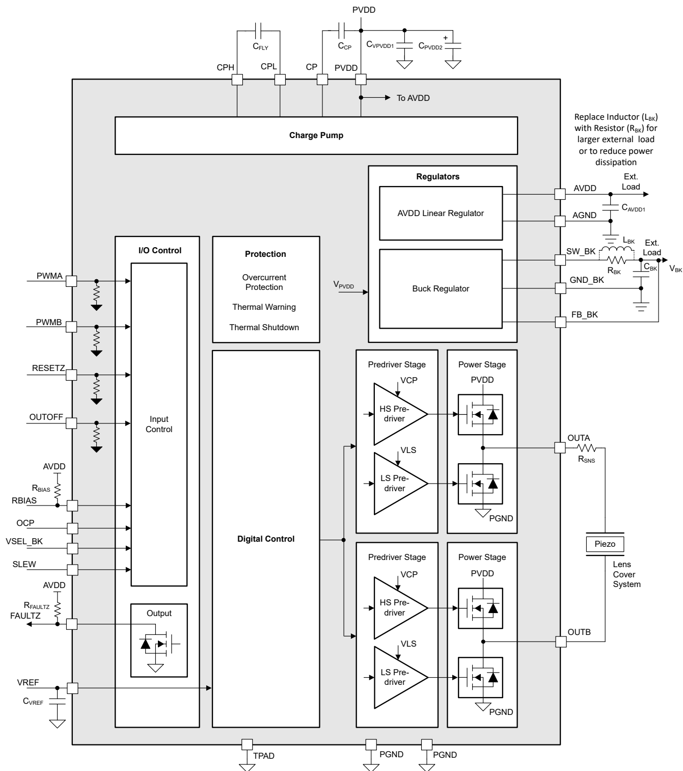
图 6-1. DRV2911-Q1 方框图
