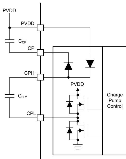
图 6-12. DRV2911-Q1 电荷泵
