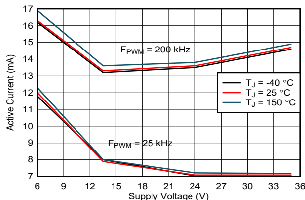
图 5-1. 电源电流与电源电压间的关系
