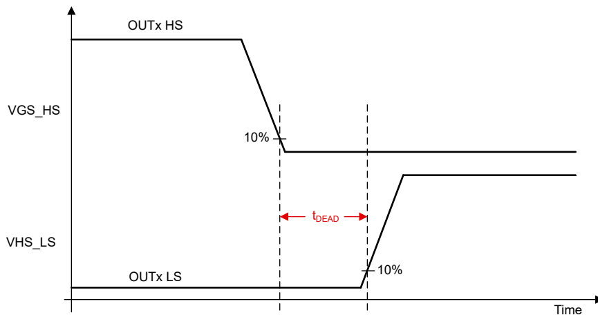
图 6-16. 死区时间
