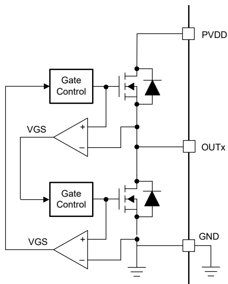
图 6-15. 跨导保护
