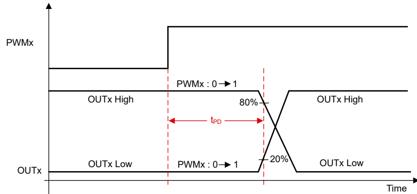
图 6-17. 传播延迟
