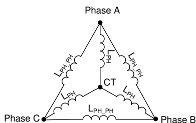
图 6-39. 电机电感
