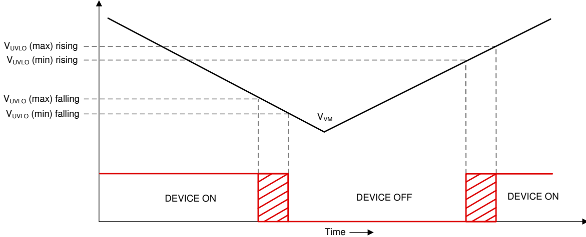
图 6-49. VM 电源欠压锁定
