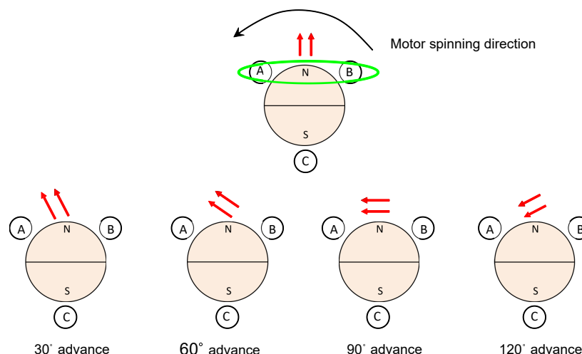
图 6-29. IPD 超前角度
