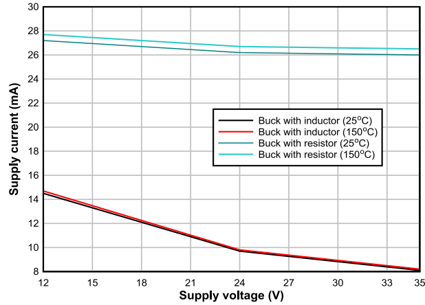
图 5-1. 电源电压两端的电源电流
