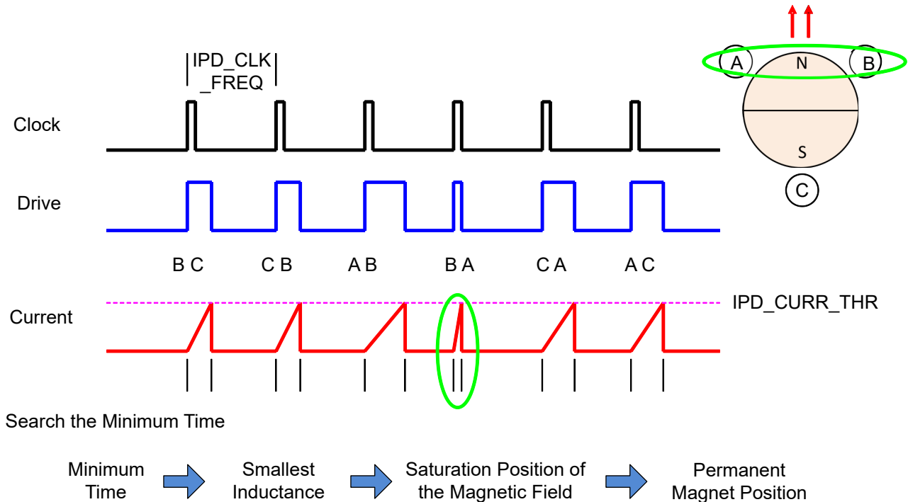
图 6-26. IPD 操作
