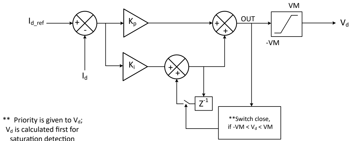
图 6-36. I_d 电流 PI 控制
