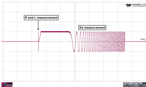
图 7-3. MPET - 相电流
