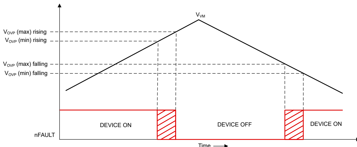
图 6-50. 过压保护
