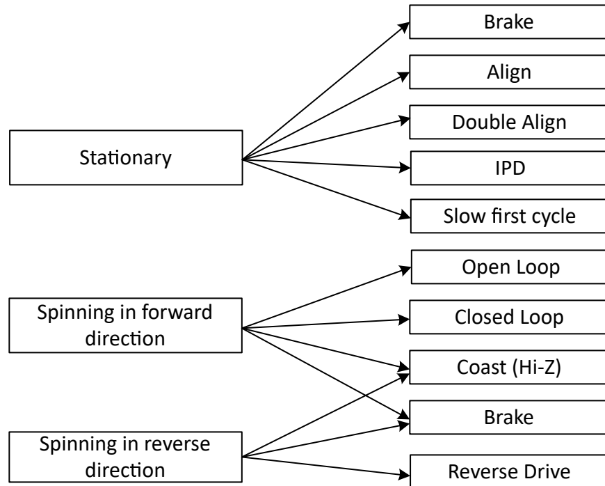
图 6-22. 在不同初始条件下启动电机
