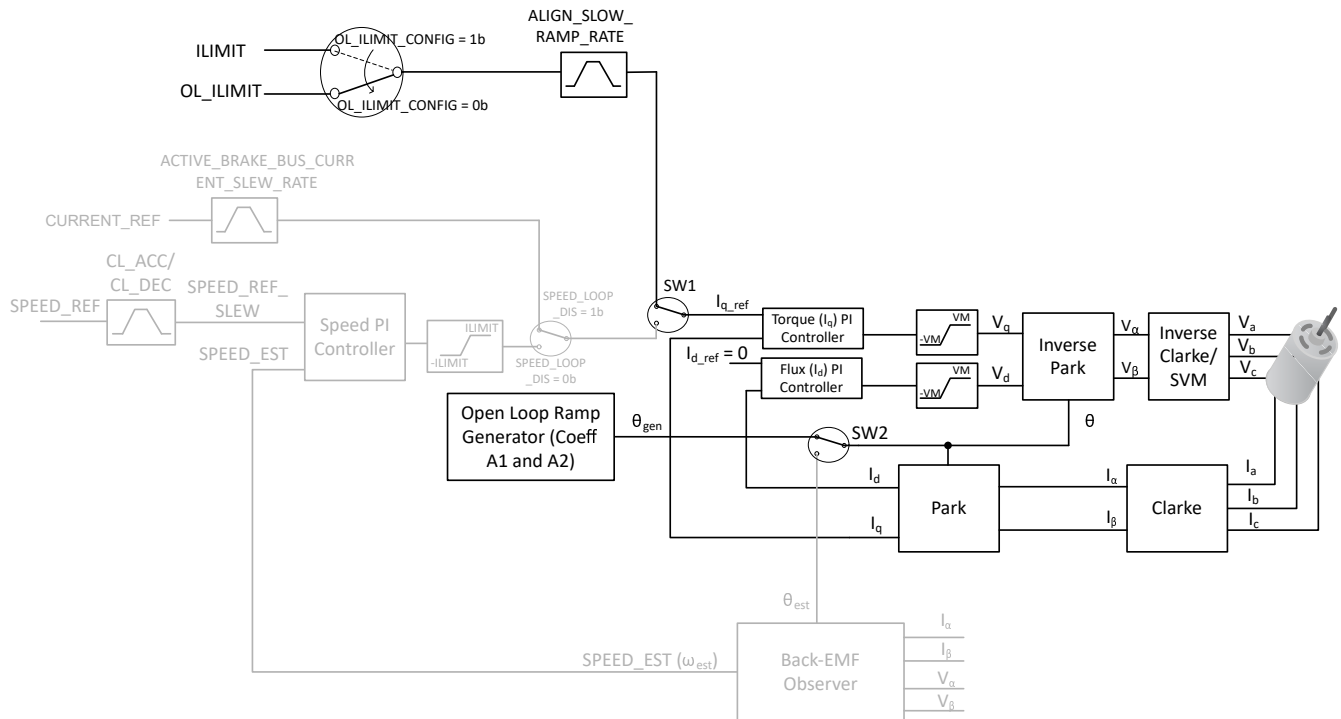
图 6-30. 开环
