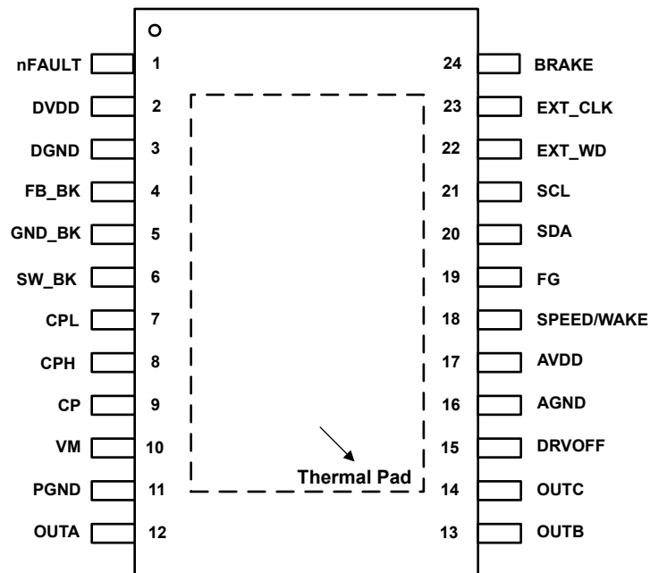
图 4-2. MCF8315C，24 引脚 HTSSOP（带有外露散热焊盘），顶视图
