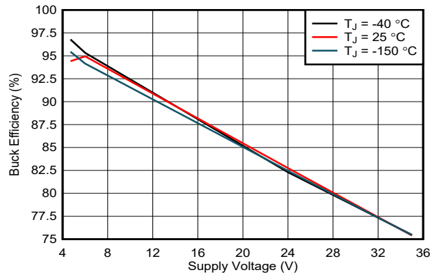
图 5-3. 降压稳压器在电源电压下的效率
