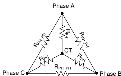
图 6-38. 电机电阻
