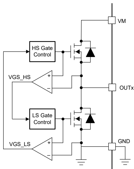
图 6-12. 跨导保护
