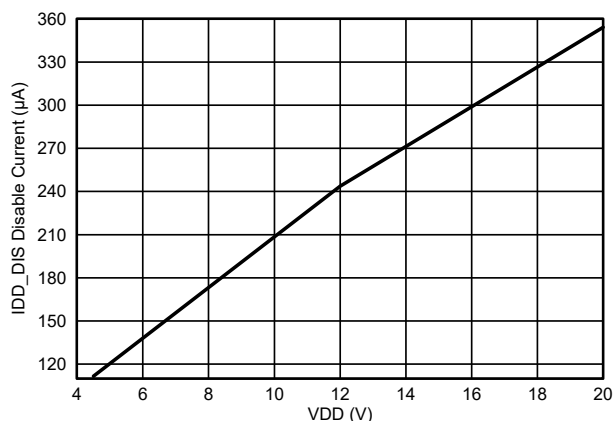
图 6-6. Disable Current
