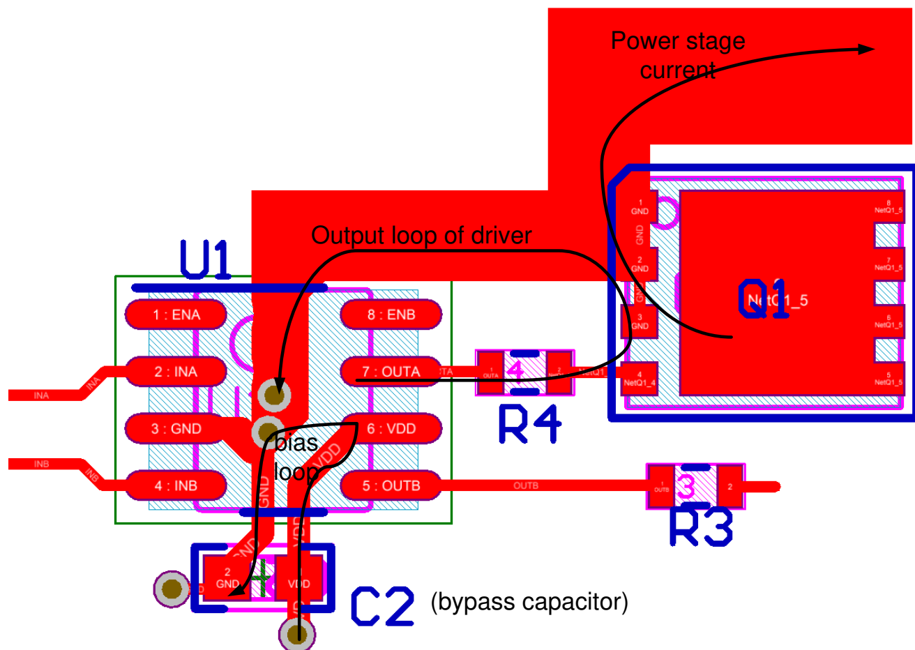
图 10-1. UCC27444-Q1 Layout Example
