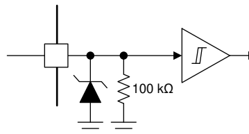
图 8-9. 逻辑电平输入
