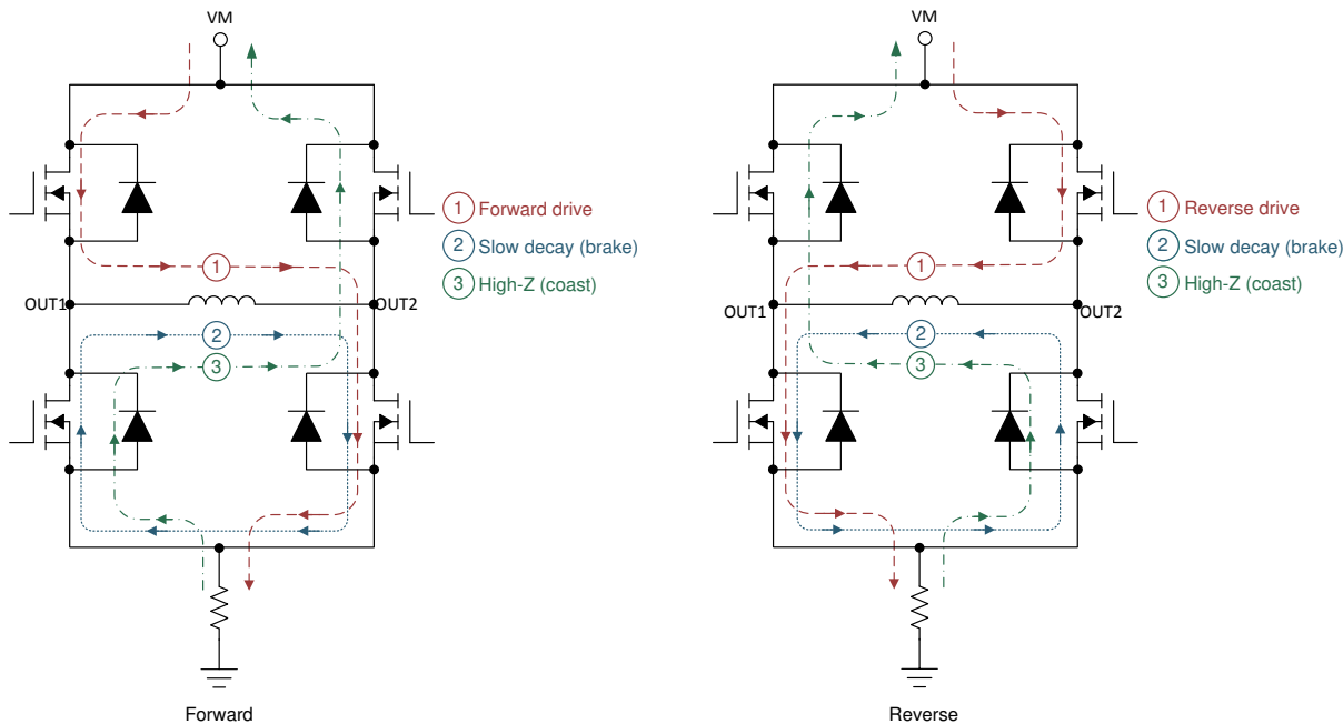
图 8-3. H 桥状态
