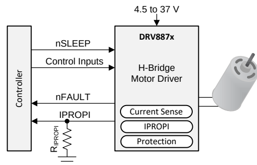
简化原理图
