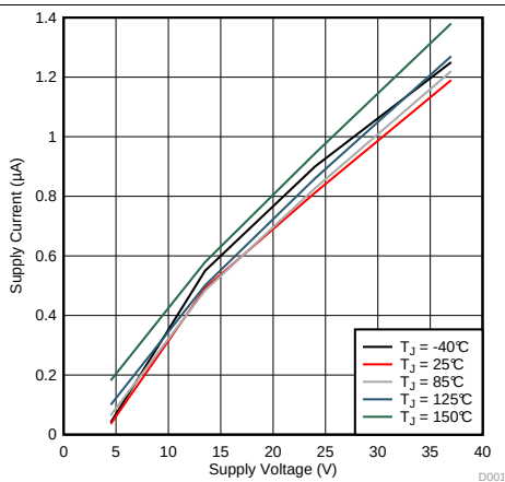
图 2. 睡眠电流 (I VMQ ) 与电源电压 (V VM )
