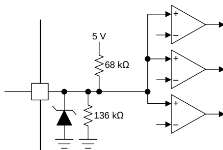
图 17. 四电平输入
