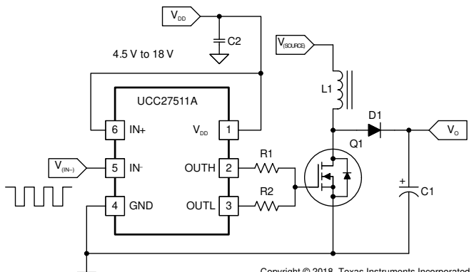
反相输入应用图
