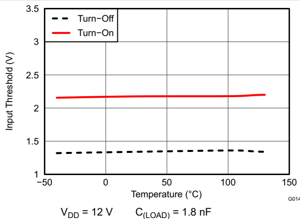
图 5-9. Input Threshold vs Temperature
