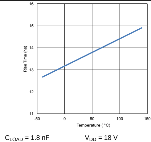
图 25. Rise Time vs. Temperature
