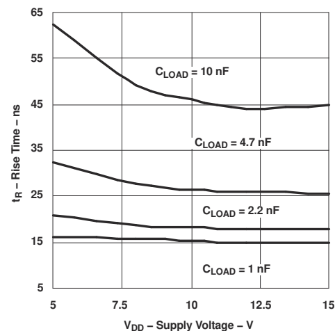
图 8-7. Rise Time vs Supply Voltage
