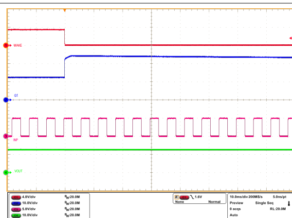
图 8-5. 由于 \overline{LPM} 为低电平，即使在唤醒后，INP 也无法控制 G1
