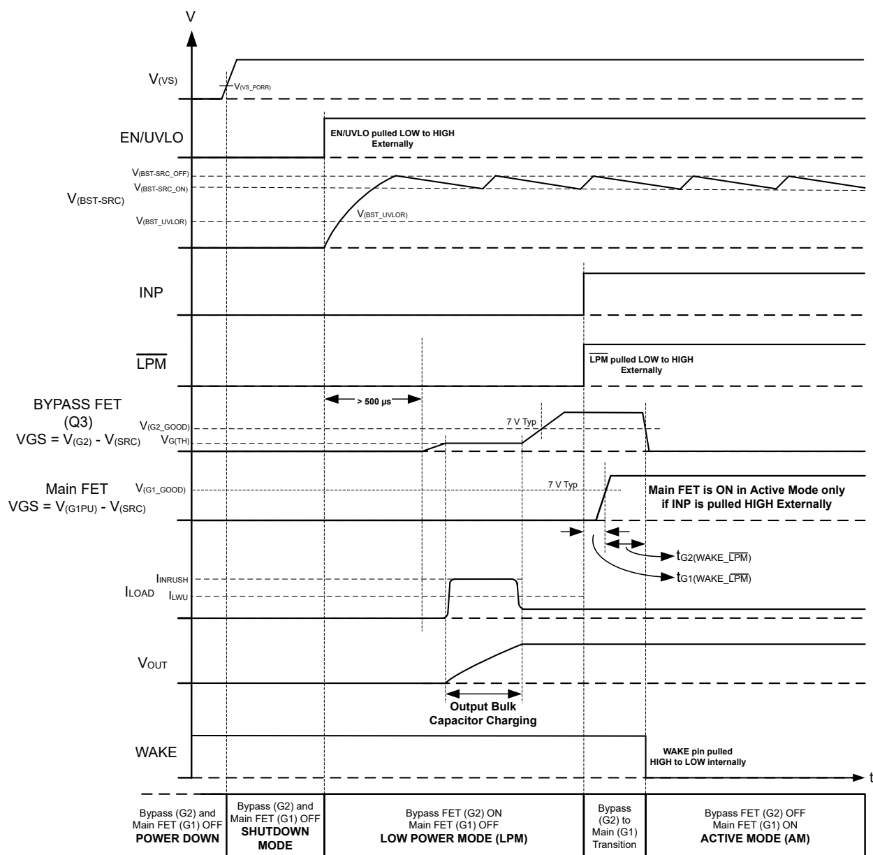
图 7-13. 包含 LPM 触发器的状态转换时序图
