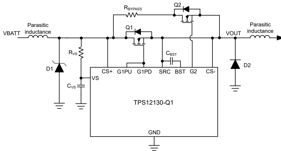
图 8-16. 采用可选保护元件的 TPS12130-Q1 电路实施方案
