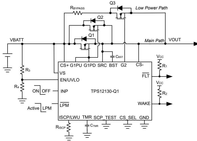
图 8-1. 使用自动负载唤醒功能来驱动全时供电 (PAAT) 负载的 TPS12130-Q1 应用电路
