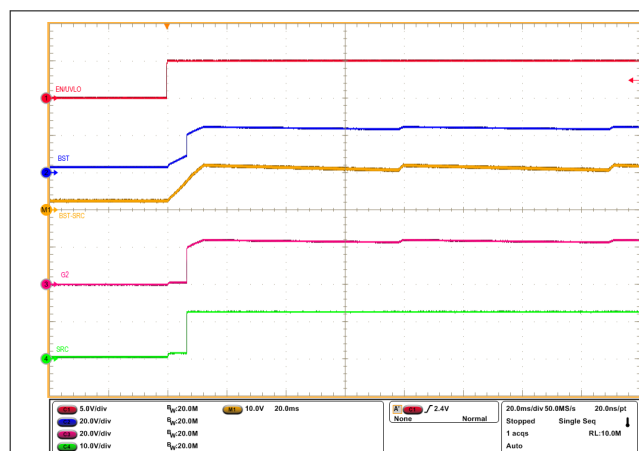
图 8-2. 低功耗路径的启动曲线 ( \overline{LPM} = 低电平， V_{IN} = 12V ，无负载， CBST = 470nF )
