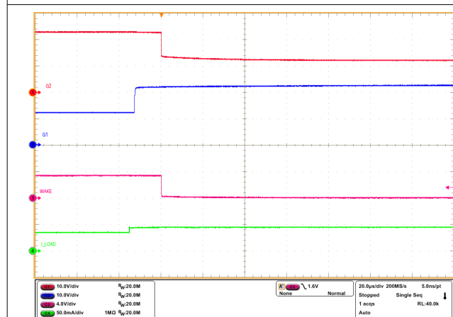
图 8-4. 从 LPM 到工作模式的状态转换放大视图 ( \overline{LPM} = 低电平， V_{IN} = 12V ， EN/UVLO = 高电平)
