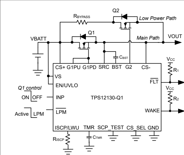
图 7-7. TPS12130-Q1 应用电路，其电流检测功能基于主 FET RDSON
