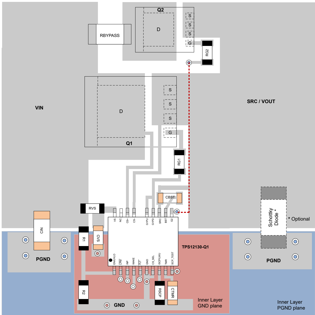
图 8-17. 具有低功耗路径的 TPS1213-Q1 典型 PCB 布局示例
