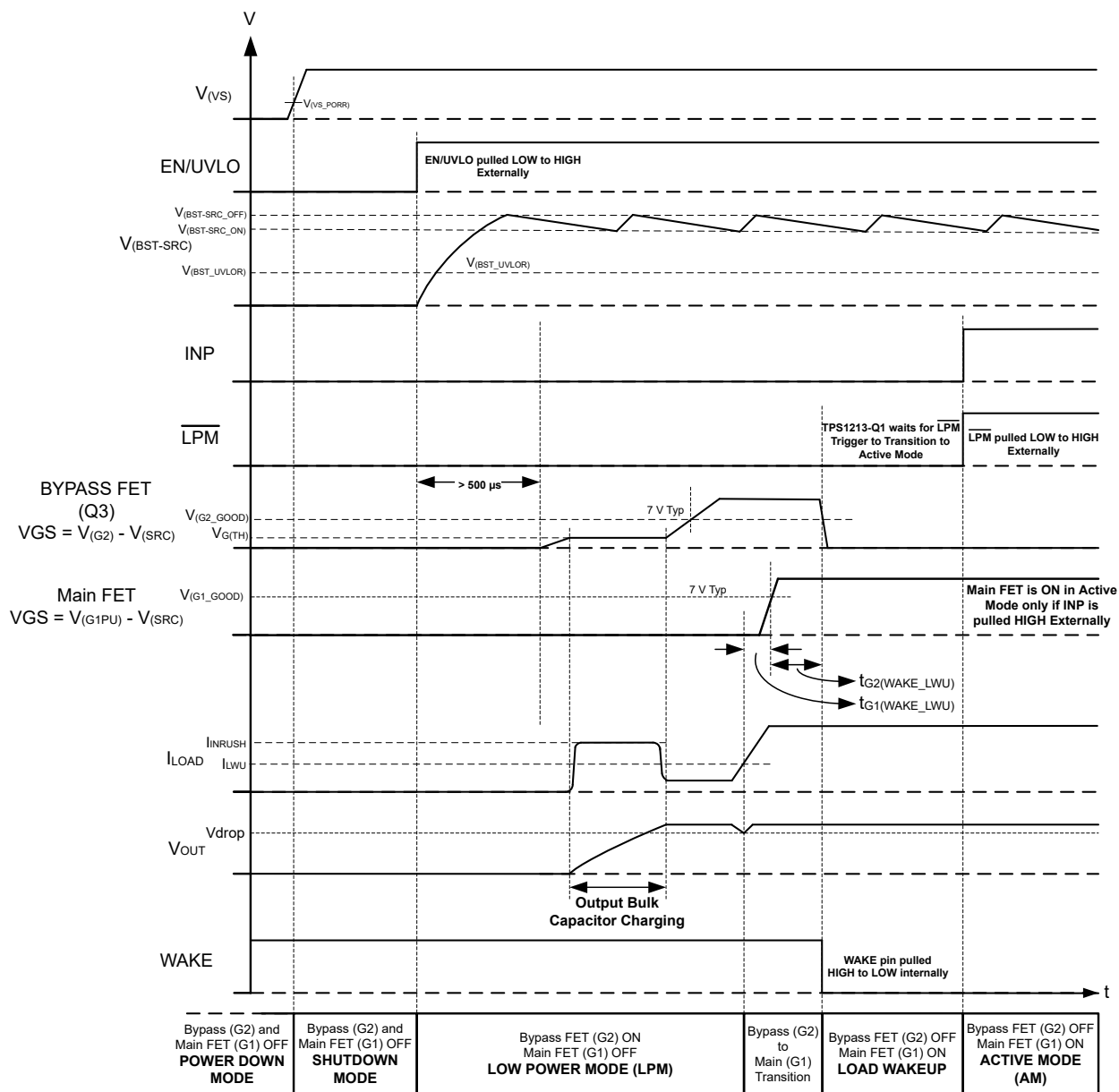
图 7-12. 包含负载唤醒事件的状态转换时序图
