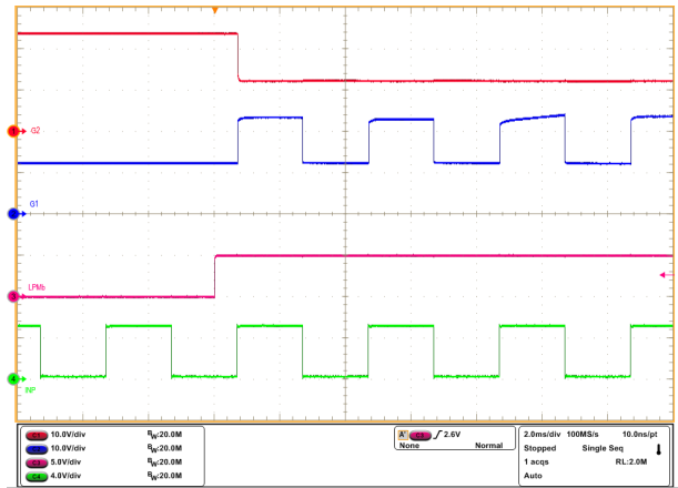
图 8-7. 当 LPM = 低电平到高电平时, INP 获得对 G1 的控制 ( VIN = 12V, 无负载 )
