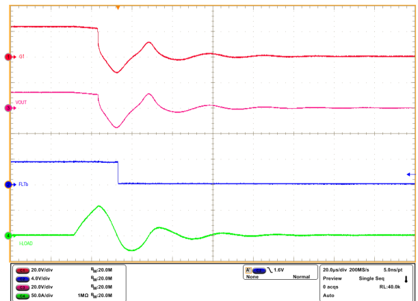
图 8-11. TPS1213-Q1 的输出短路响应
