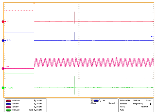
图 8-9. TPS1213-Q1 针对过流故障的自动重试响应
