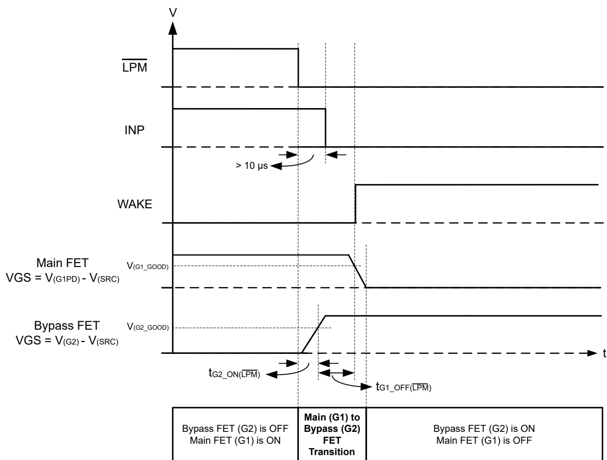
图 7-14. 从工作模式进入低功耗模式的 \overline{\text{LPM}} 和 \text{INP} 信号时序控制注意事项
