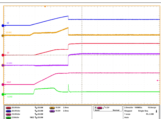
图 8-14. 输出端为 220\mu\text{F} 且负载为 0.5\text{A} 时的浪涌电流曲线 ( \overline{\text{LPM}} = 低电平 )
