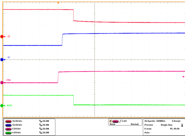
图 8-6. 从 LPM 到工作模式的状态转换 ( LPM = 低电平到高电平, VIN = 12V, 无负载 )
