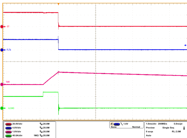
图 8-8. TPS1213-Q1 EVM 在 40A 至 55A 负载阶跃下的过流响应
