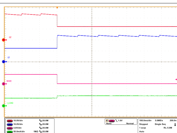
图 8-3. 从 LPM 到工作模式的状态转换 ( \overline{LPM} = 低电平， V_{IN} = 12V ， EN/UVLO = 高电平)
