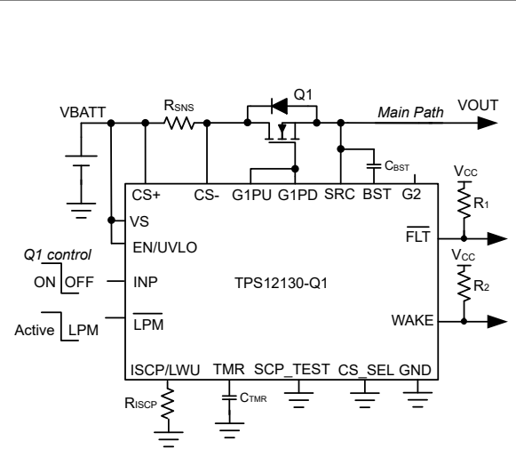
图 7-8. TPS12130-Q1 应用电路，其电流检测功能基于外部检测电阻 R_{SNS}
