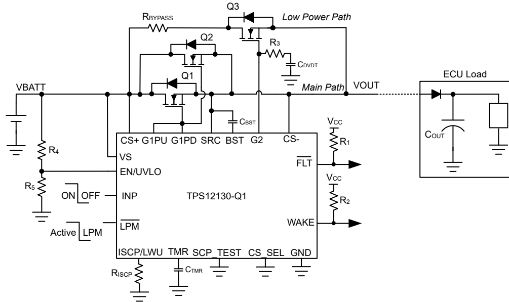
图 8-12. 使用自动负载唤醒和输出大容量电容器充电功能来驱动全时供电 (PAAT) 负载的 TPS1213-Q1 应用电路
