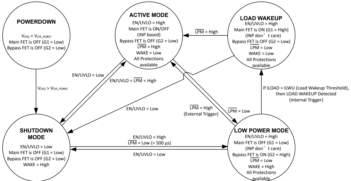
图 7-11. TPS12130-Q1 状态图
