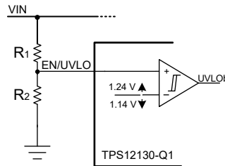
图 7-15. 欠压保护阈值编程
