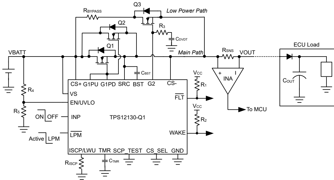
图 8-15. 具有双向电流检测和软件 I2t 的常开型汽车级电子保险丝
