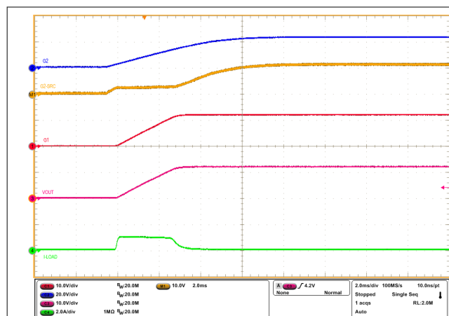
图 8-13. 输出端为 220\mu\text{F} 时的浪涌电流曲线 ( \overline{\text{LPM}} = 低电平 )
