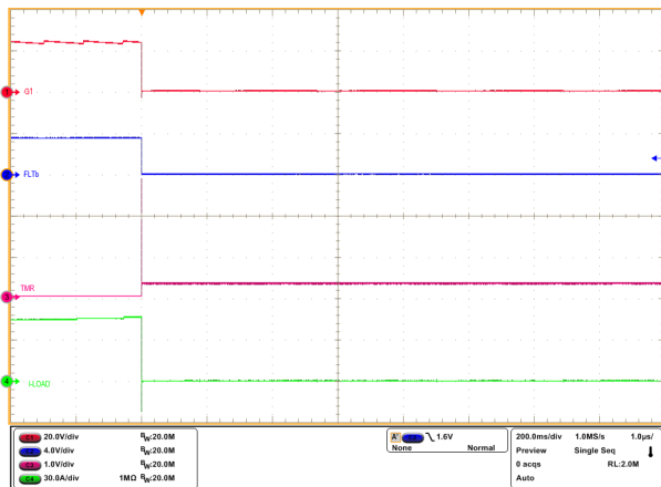
图 8-10. TPS1213-Q1 针对过流故障的闭锁响应
