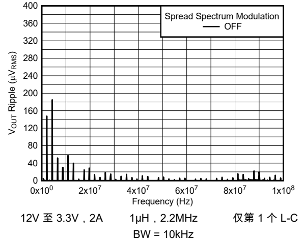
图 5-10. 第 1 个 L-C 滤波器之后的 V_{OUT} 纹波 FFT
