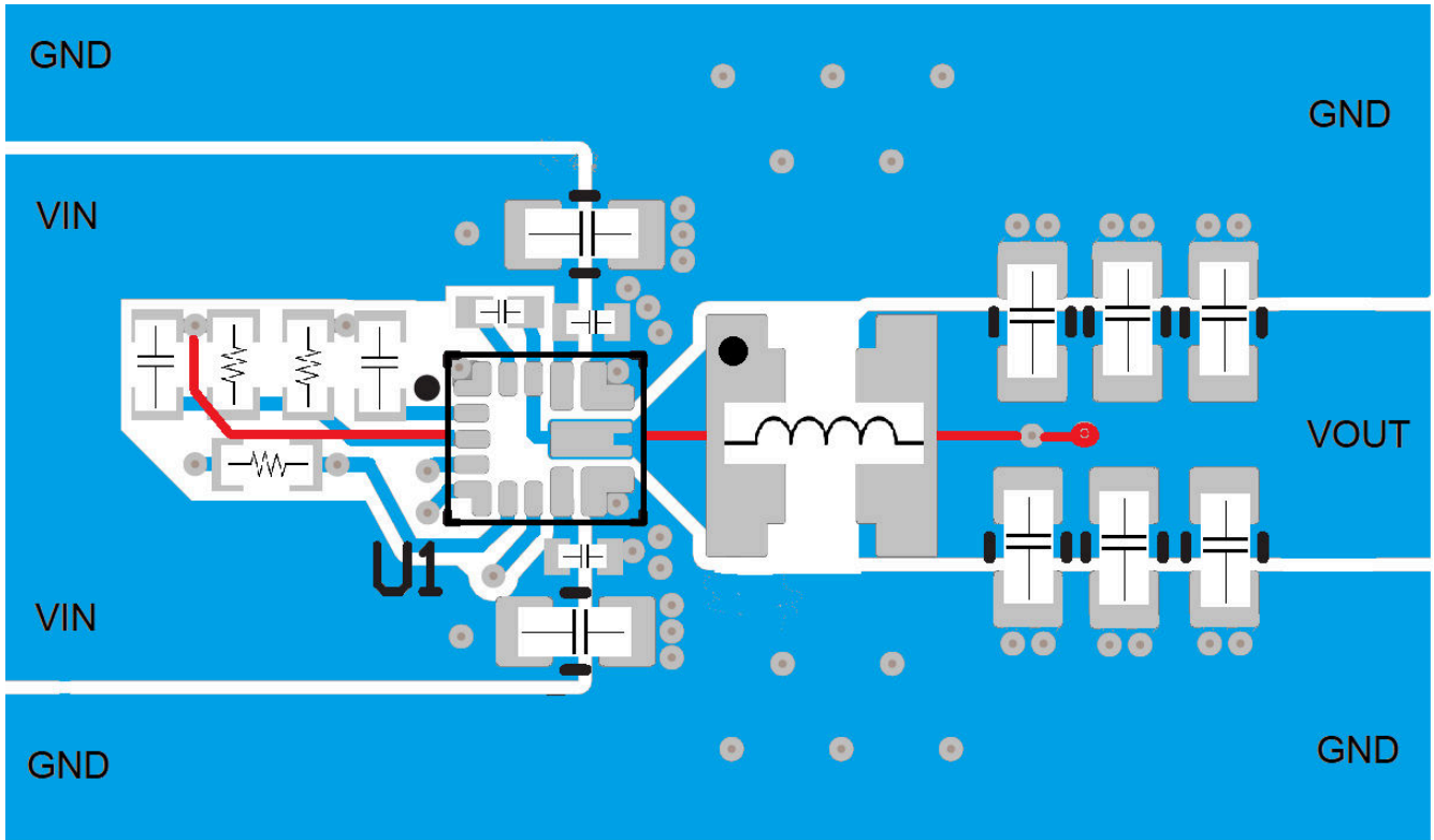
图 7-2. 单个 L-C 滤波器的建议布局
