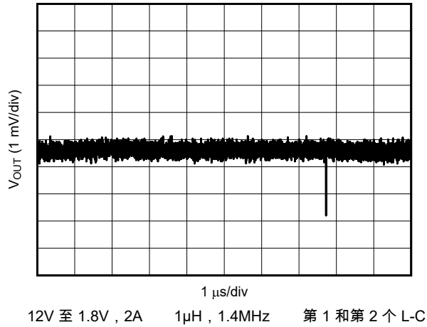
图 5-7. 第 2 个 L-C 滤波器之后的 V_{OUT} 纹波
