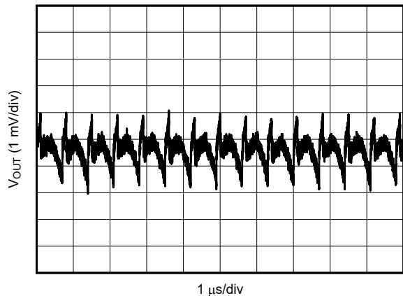
图 5-3. 第 2 个 L-C 滤波器之后的 V_{OUT} 纹波
