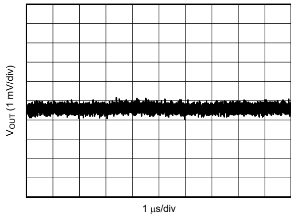
图 5-1. 第 1 个 L-C 滤波器之后的 V_{OUT} 纹波
