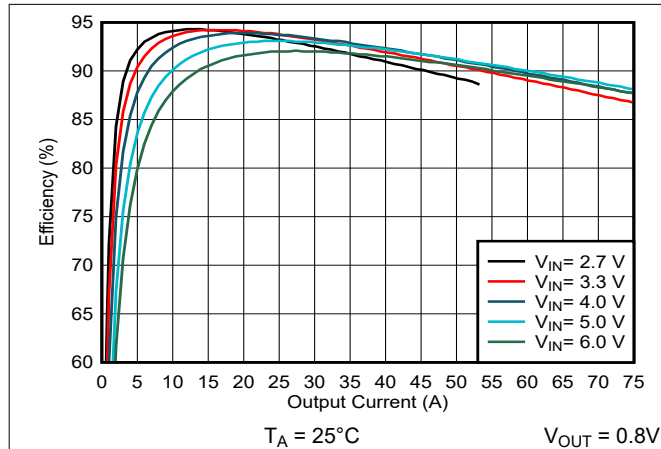
图 9-36. 效率与输出电流间的关系
