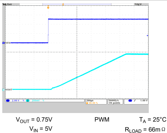
图 9-20. 启动时序
