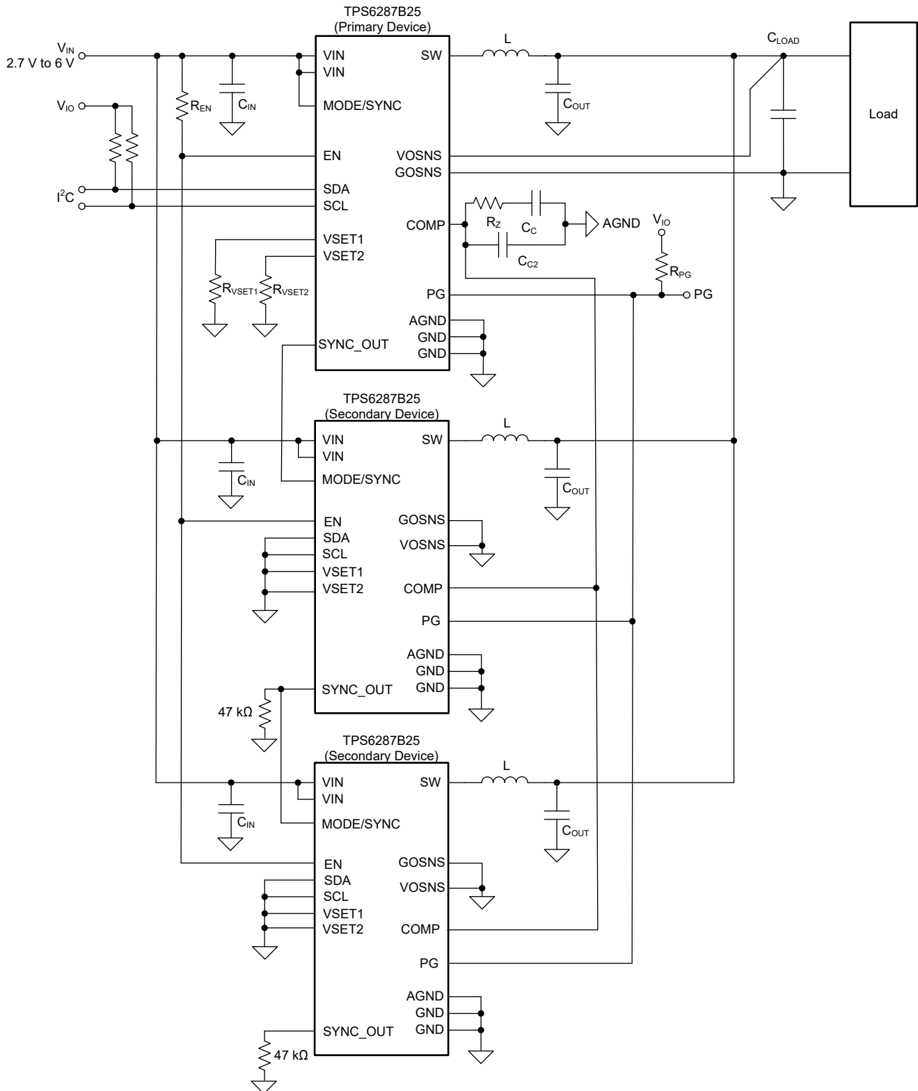
图 9-35. 堆叠三个器件
