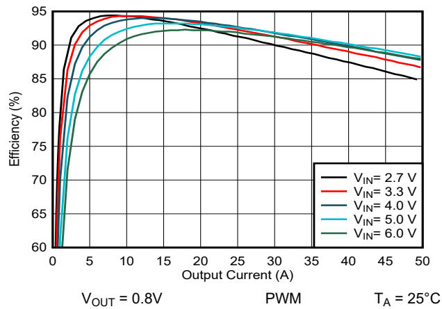
图 9-27. 效率与输出电流间的关系
