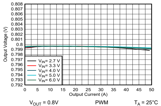
图 9-28. 输出电压与输出电流间的关系
