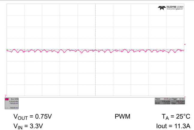
图 9-21. 输出电压纹波
