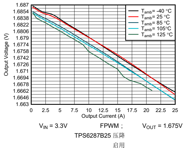
图 9-19. 输出电压与输出电流间的关系
