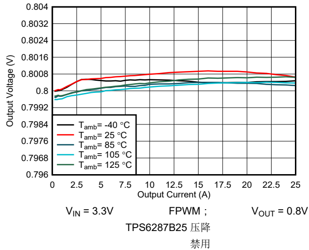
图 9-16. 输出电压与输出电流间的关系
