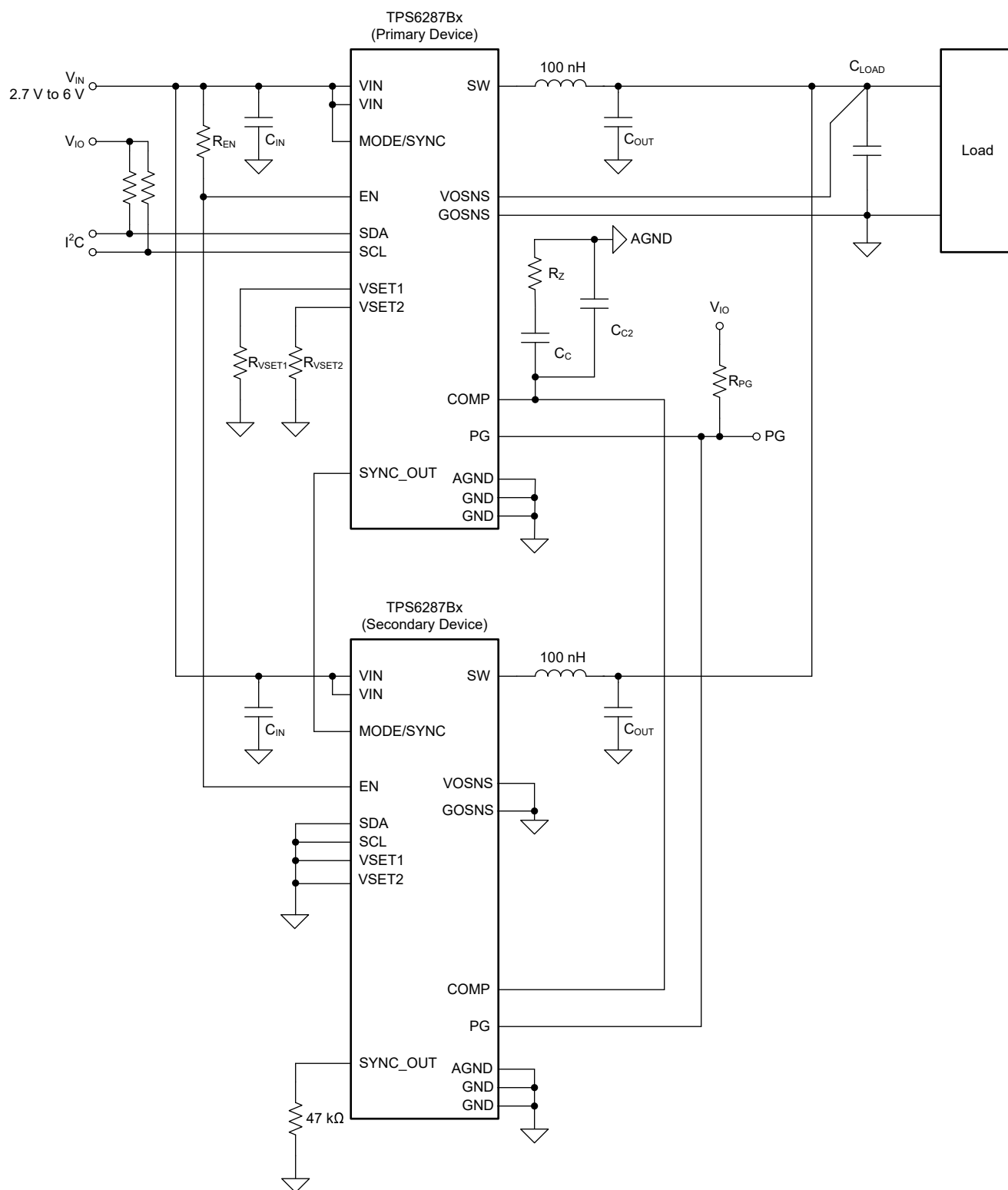
图 9-26. 堆叠两个器件，电流高达 50A
