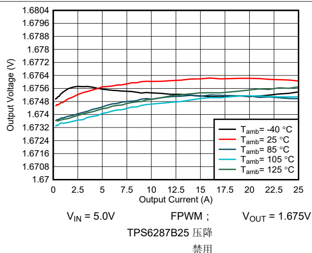
图 9-12. 输出电压与输出电流间的关系
