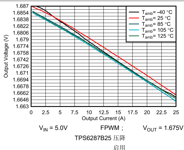
图 9-13. 输出电压与输出电流间的关系
