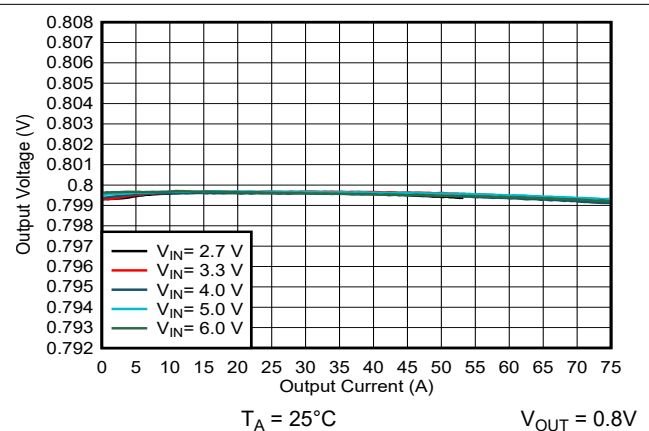
图 9-37. 输出电压与输出电流间的关系
