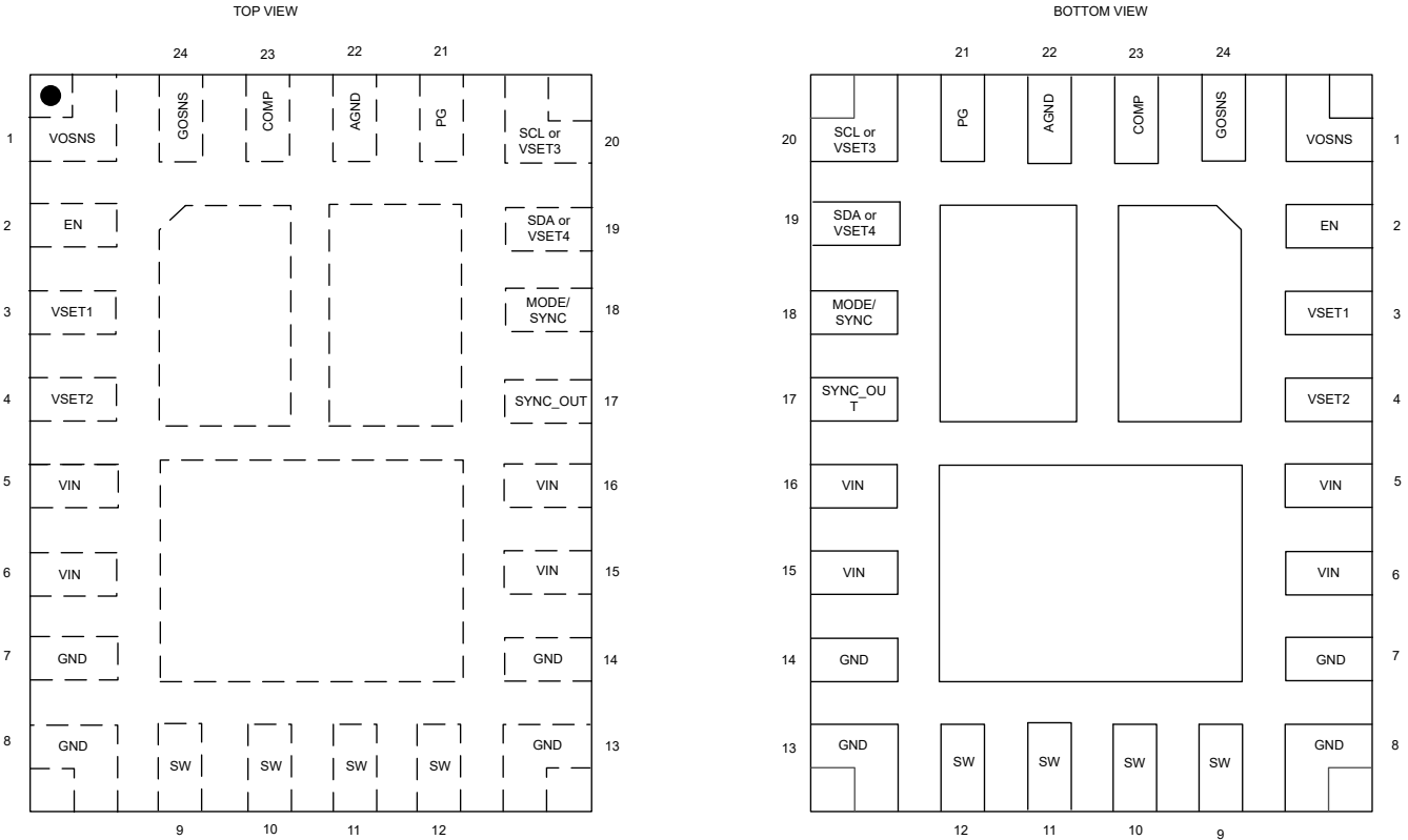
图 5-1. RZV 封装 24 引脚 VQFN
