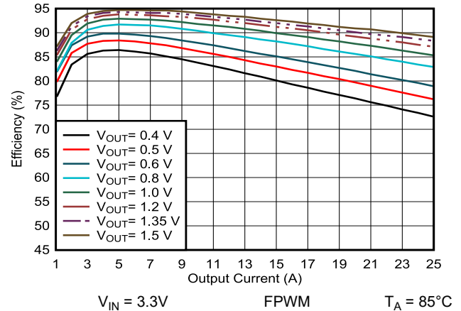
图 9-5. 效率与输出电流间的关系
