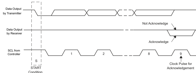
图 8-18. I 2 C 总线上的确认
