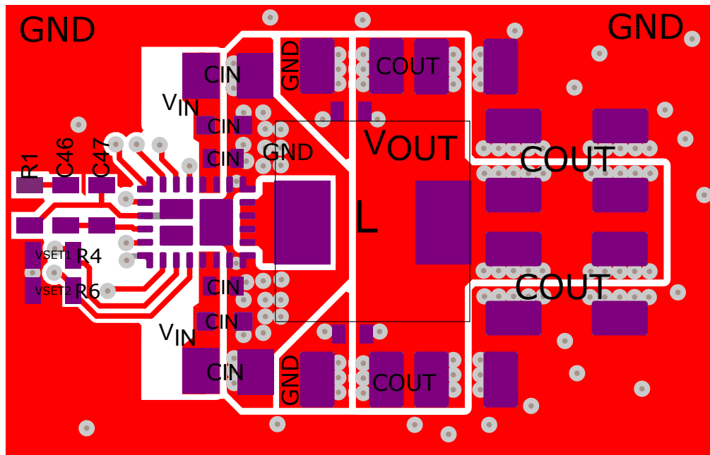
图 9-40. TPS6287B25 EVM 顶层
