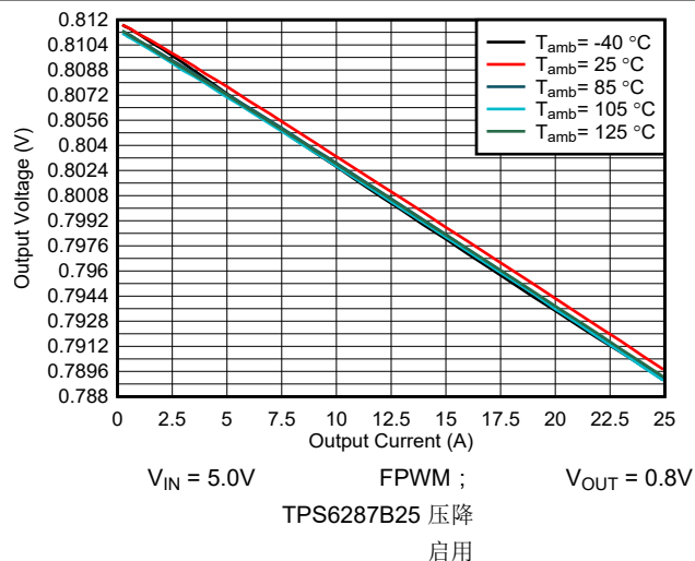
图 9-11. 输出电压与输出电流间的关系
