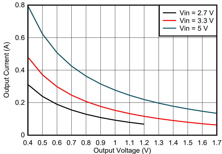
图 8-5. f_{sw} = 1.5\text{MHz} 时的输出电流 PFM-DCM 进入阈值
