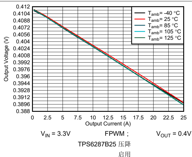
图 9-15. 输出电压与输出电流间的关系
