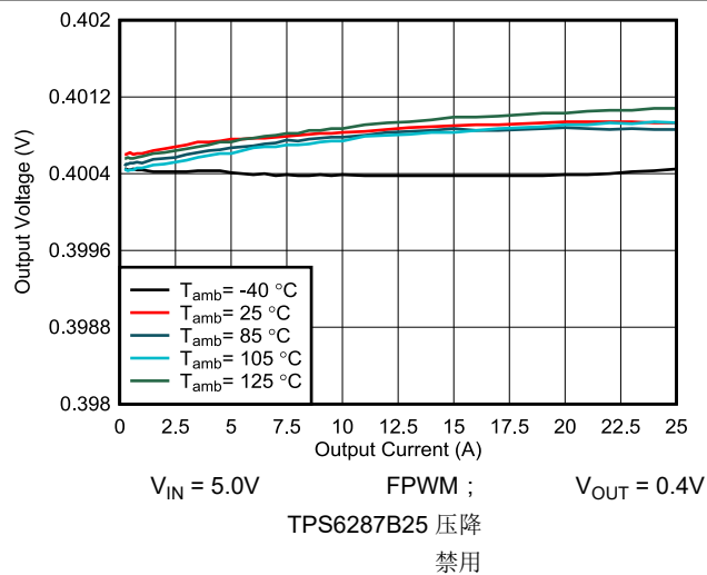
图 9-8. 输出电压与输出电流间的关系
