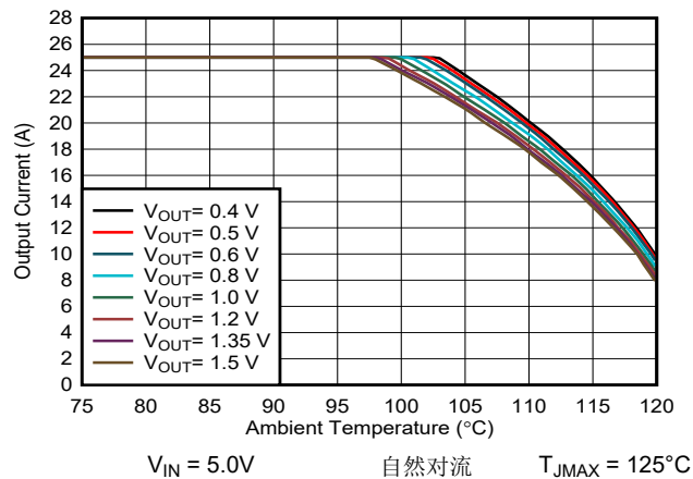
图 9-6. 安全操作区域
