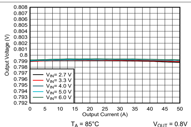
图 9-39. 输出电压与输出电流间的关系
