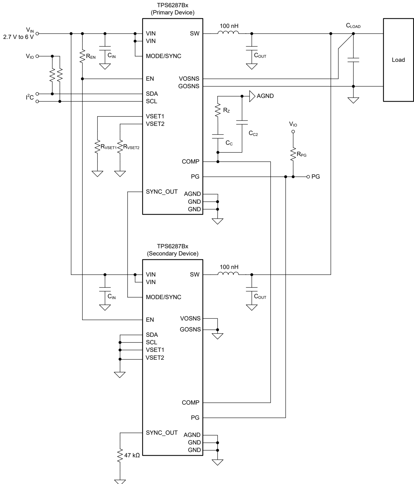
图 8-15. 堆叠配置中的两个 TPS6287Bx 器件
