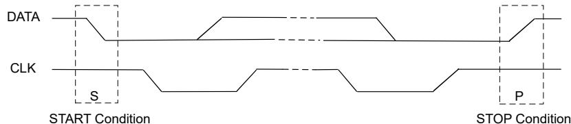
图 8-16. START 和 STOP 条件
