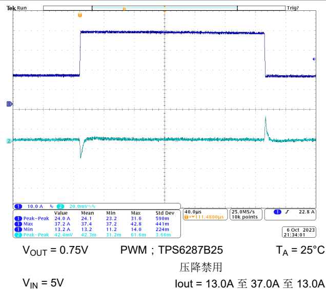
图 9-31. 负载瞬态响应
