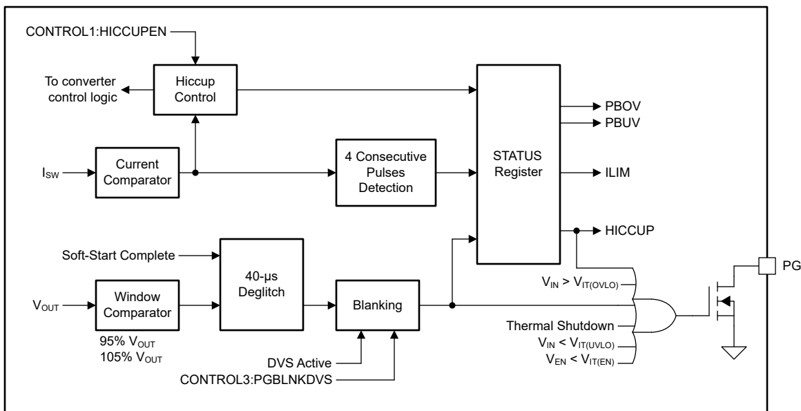
图 8-13. 电源正常状态指示功能方框图 (独立/主器件)
