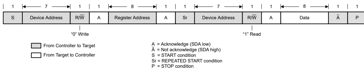
图 8-21. 标准-、快速、快速+ 模式下的“读取”数据传输格式
