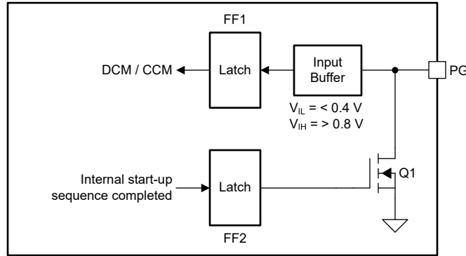
图 8-14. 电源正常状态指示功能方框图 (辅助器件)
