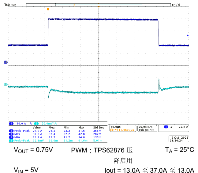
图 9-32. 负载瞬态响应
