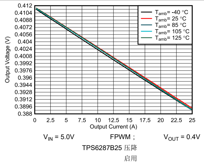
图 9-9. 输出电压与输出电流间的关系
