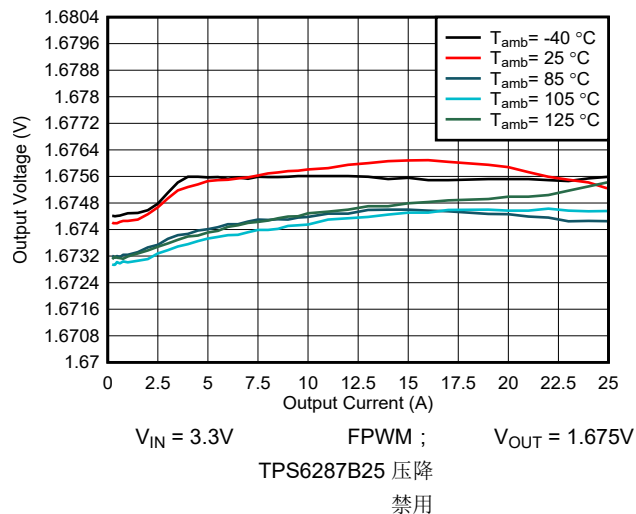
图 9-18. 输出电压与输出电流间的关系
