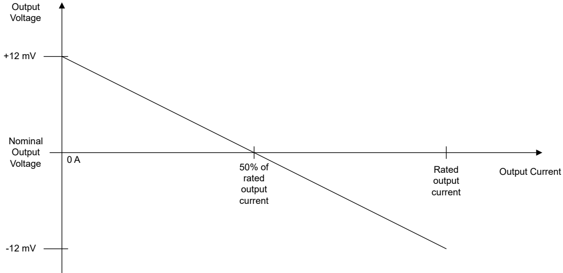
图 8-10. 电压随输出电流的调节
