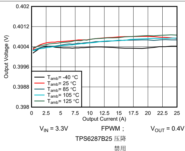
图 9-14. 输出电压与输出电流间的关系
