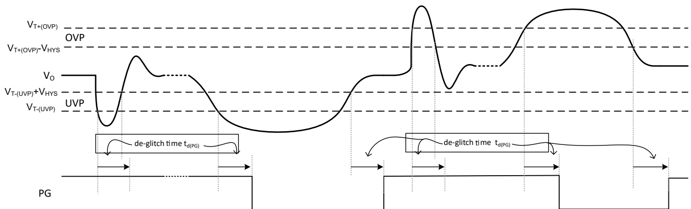
图 8-12. PG 时序
