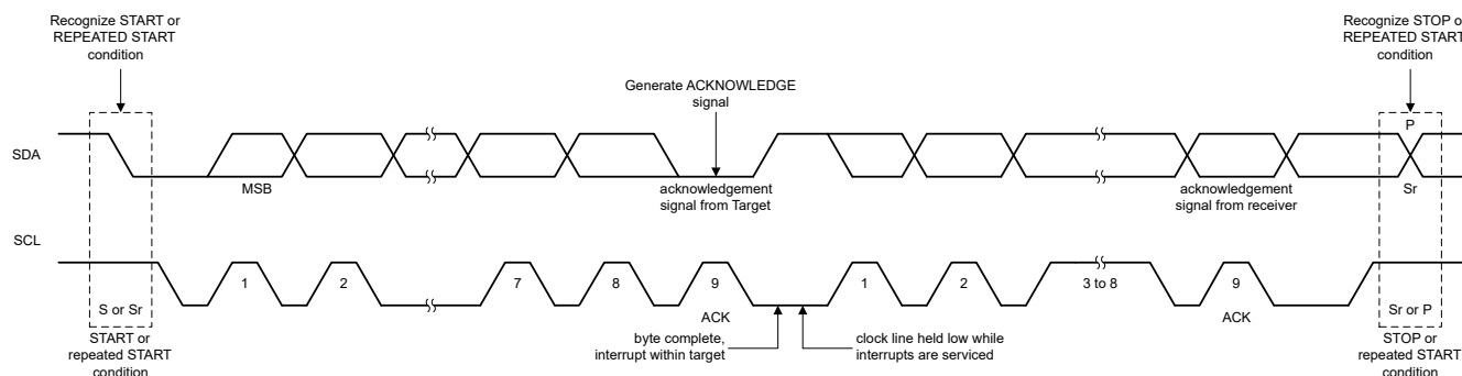
图 8-19. 总线协议
