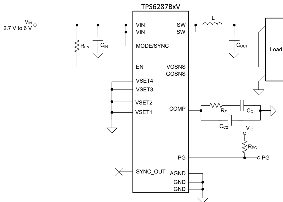
图 9-25. TPS6287BxV 的典型应用原理图
