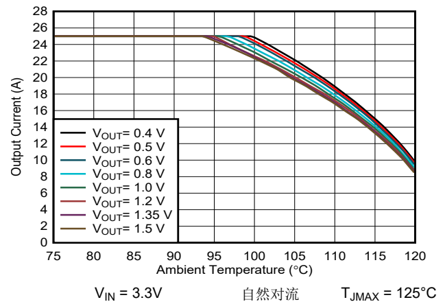
图 9-7. 安全操作区域
