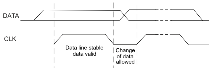
图 8-17. 串行接口上的位传输
