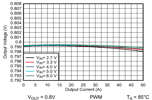
图 9-30. 输出电压与输出电流间的关系
