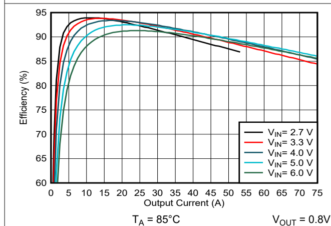
图 9-38. 效率与输出电流间的关系
