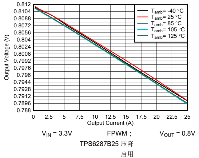
图 9-17. 输出电压与输出电流间的关系
