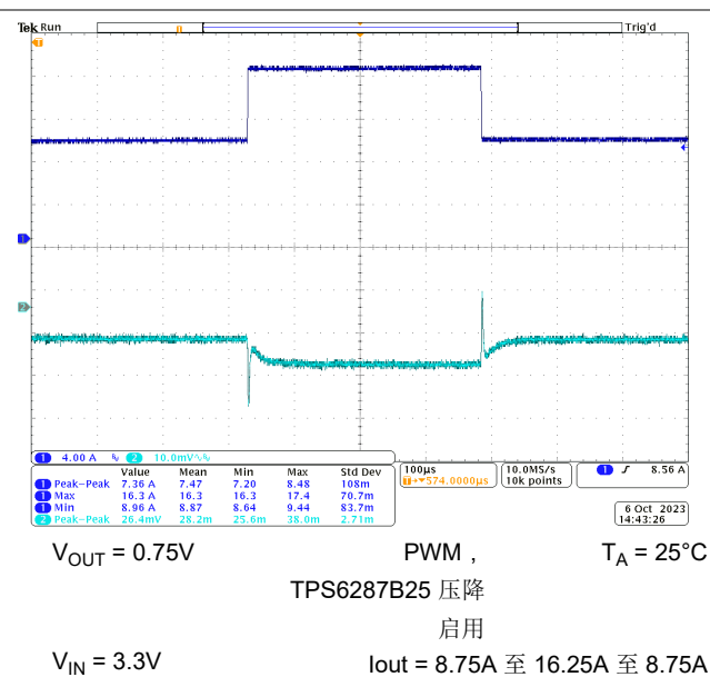
图 9-23. 负载瞬态响应
