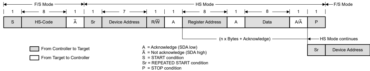
图 8-22. HS 模式下的数据传输格式
