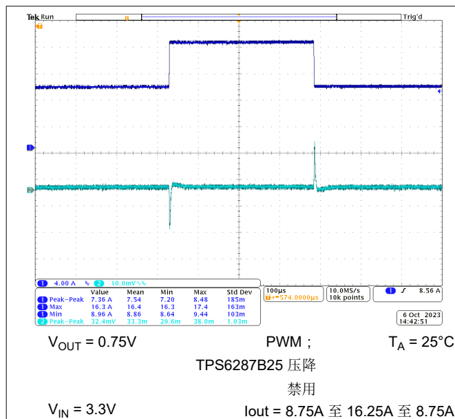
图 9-22. 负载瞬态响应
