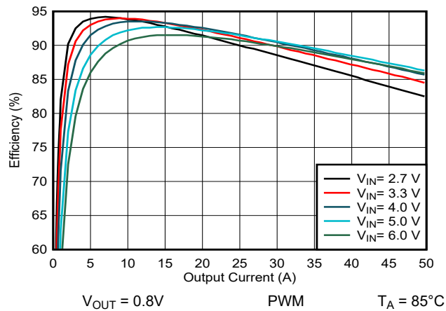
图 9-29. 效率与输出电流间的关系
