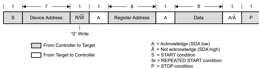
图 8-20. : 标准-、快速和快速+ 模式下的“写入”数据传输格式
