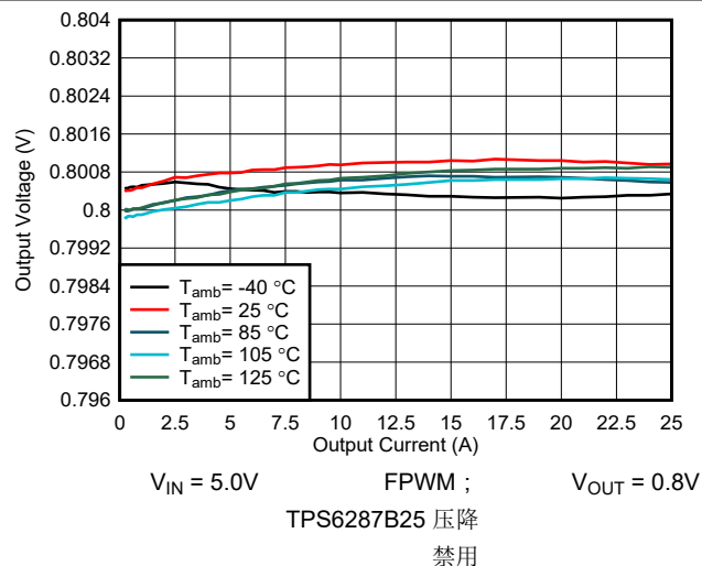
图 9-10. 输出电压与输出电流间的关系
