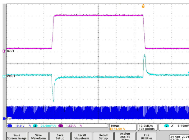
图 7-15. 负载瞬态
