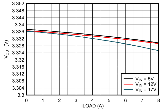
图 7-9. 输出电压与负载电流间的关系
