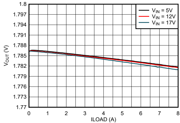
图 7-8. 输出电压与负载电流间的关系
