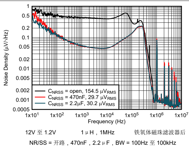
图 5-14. 输出噪声密度与频率间的关系
