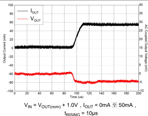
图 5-11. 负载瞬态
