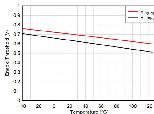
图 5-10. 使能逻辑阈值与温度间的关系
