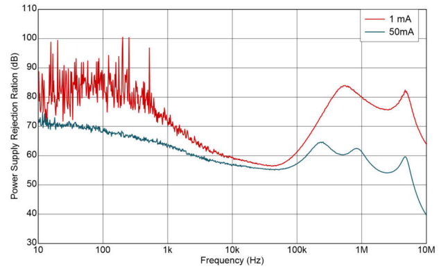
图 5-14. PSRR 与频率间的关系
