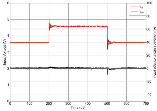
图 5-13. 线路瞬态
