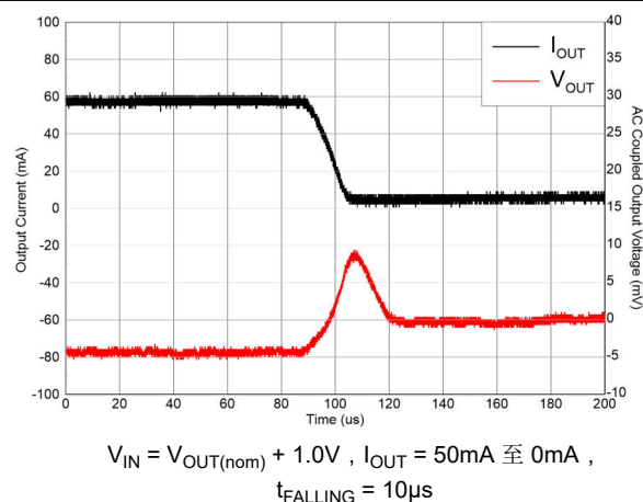
图 5-12. 负载瞬态
