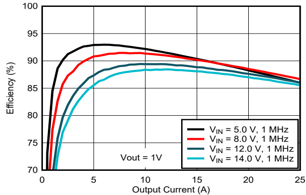
图 7-4. 效率曲线
