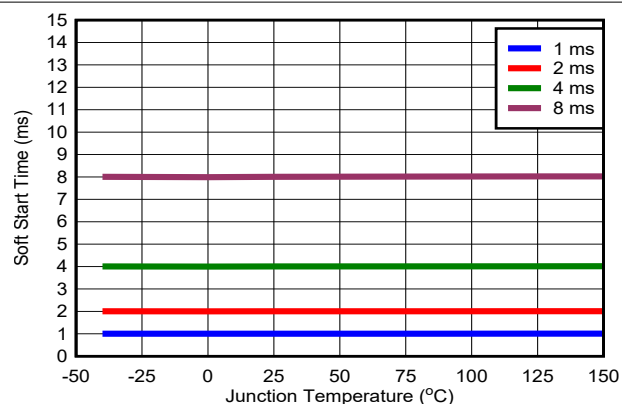
图 5-12. 软启动
