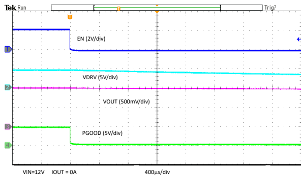
图 7-11. EN 关断
