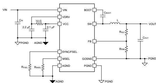
TPS543B25T 简化版应用
