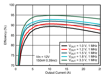
典型应用效率
