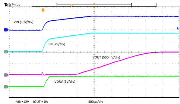
图 7-9. EN 启动 - 测量 BP5
