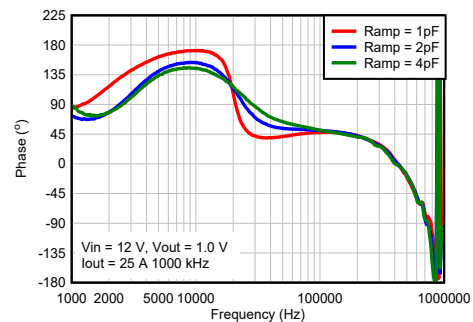
图 6-8. 环路相位与斜坡设置
