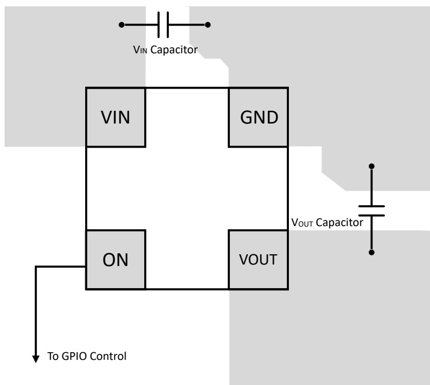
图 10-4. TPS22991 布局
