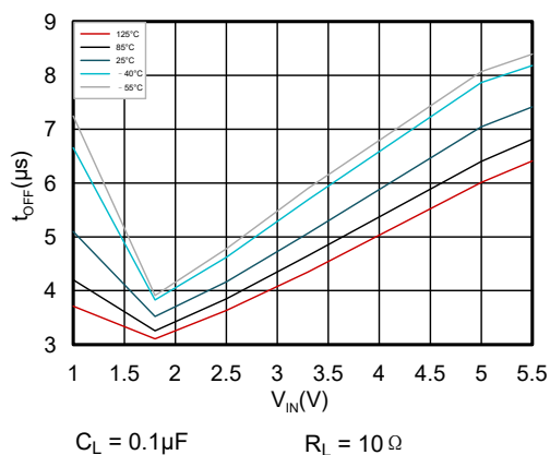
图 7-7. 关断时间与输入电压间的关系
