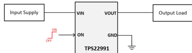
TPS22991 典型应用
