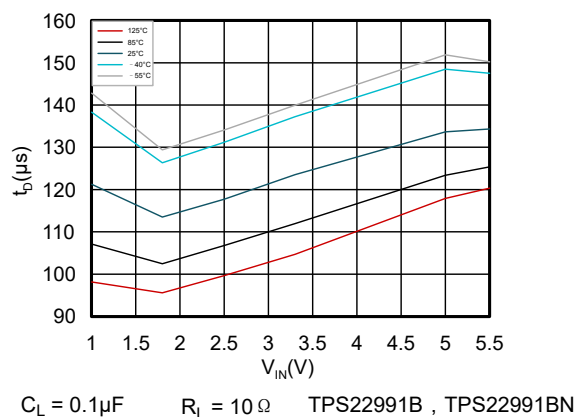
图 7-10. 延迟时间与输入电压间的关系
