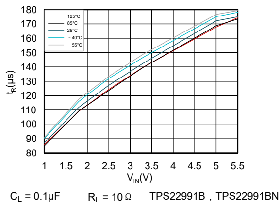
图 7-8. 上升时间与输入电压间的关系
