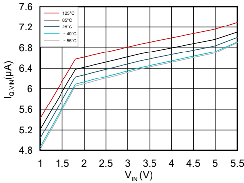
图 7-1. V_{IN} 静态电流与输入电压间的关系
