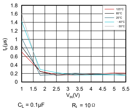
图 7-9. 下降时间与输入电压间的关系
