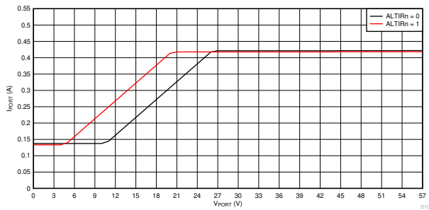
图 8-2. 浪涌期间折返 (端口开启时) : I_{LIM} 与 V_{port} 间的关系
