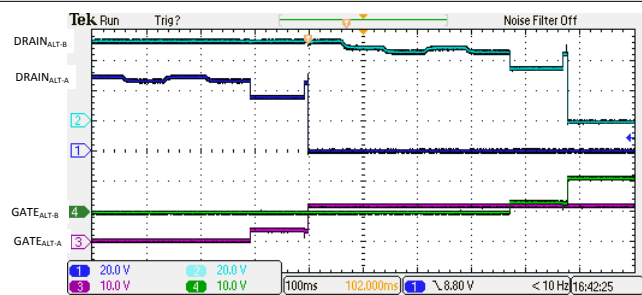
图 9-25. 4 线对双特征 1 级侦测分级和开启
