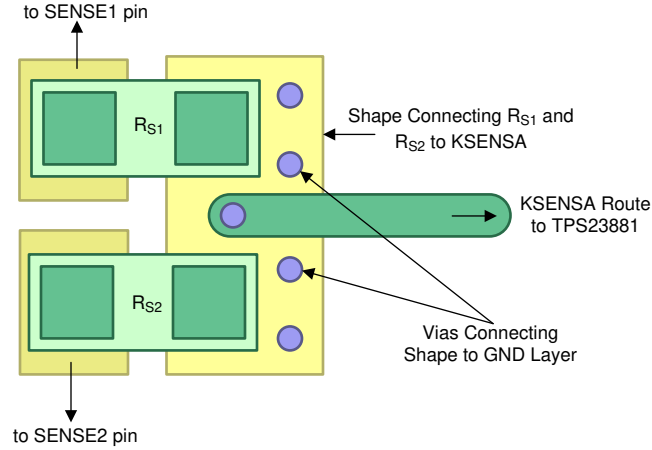
图 9-29. 开尔文检测布局示例
