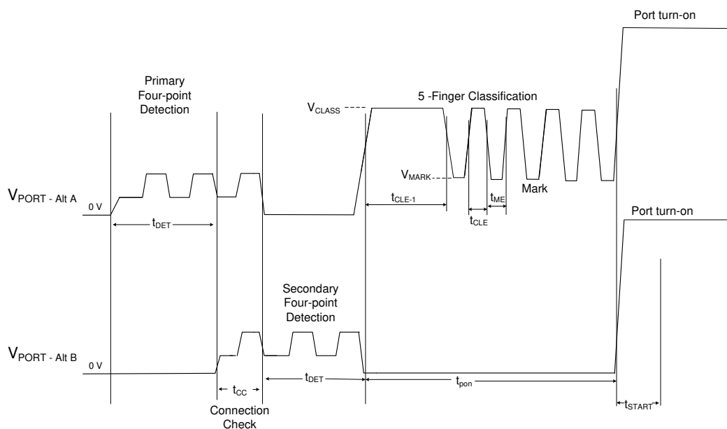
图 7-6. 4 线对单一特征检测、5 事件分级和开启
