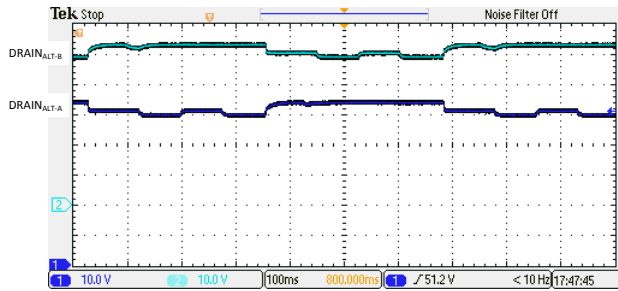
图 9-12. 4 线对低电阻 (11k \Omega ) 检测特征
