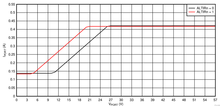
图 8-81. 浪涌折返曲线， I_{PORT} 与 V_{PORT} 间的关系
