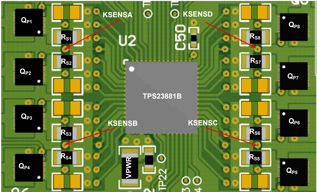
图 9-30. 八端口布局示例 (顶部)
