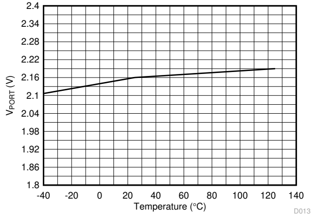
图 6-13. 电源正常阈值与温度间的关系
