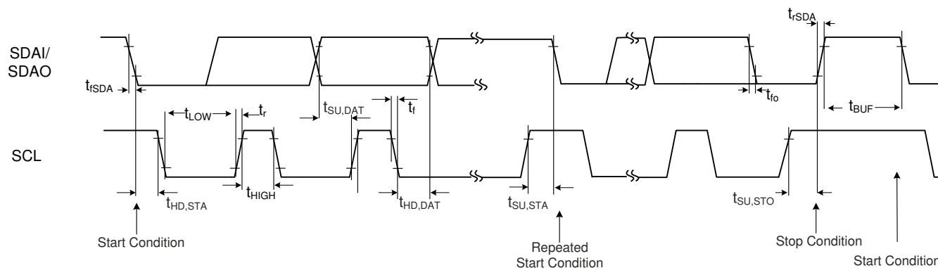
图 7-1. I 2 C 时序
