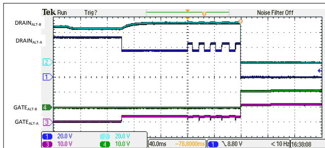
图 9-22. 4 线对单一特征 5 级侦测分级和开启
