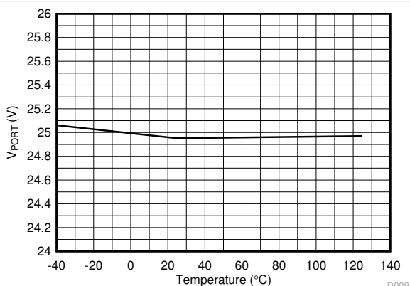
图 6-9. 发现开路电压与温度间的关系
