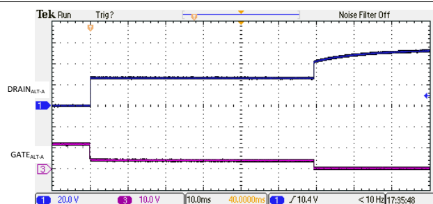
图 9-4. 2 线对 I_{LIM} 折返和关闭
