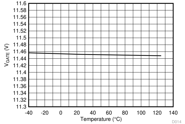
图 6-14. 栅极电压 (端口开启) 与温度间的关系
