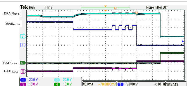
图 9-21. 4 线对单一特征 4 级侦测分级和开启
