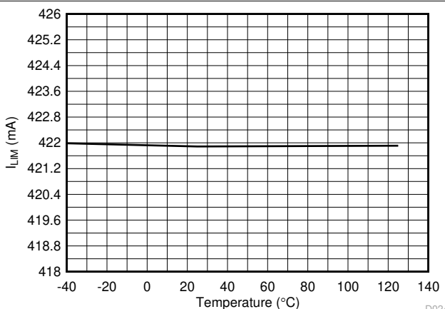
图 6-24. 1x 模式 (2xFBn = 0) 电流限制与温度间的关系
