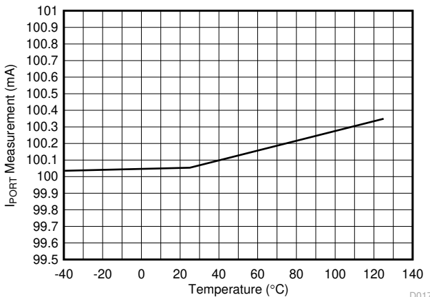
图 6-17. 端口电流 ADC 测量值 (100mA) 与温度间的关系
