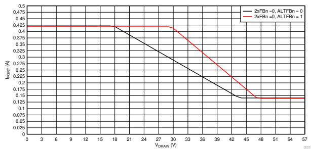
图 8-79. 1x 模式 (2xFBn = 0) 折返曲线， I_{PORT} 与 V_{DRAIN} 间的关系
