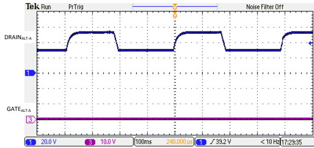
图 9-10. 2 线对开路检测特征
