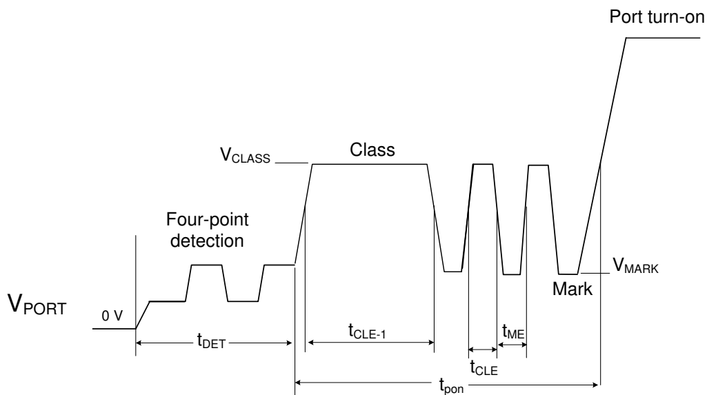
图 7-4. 2 线对检测、3 事件分级和开启
