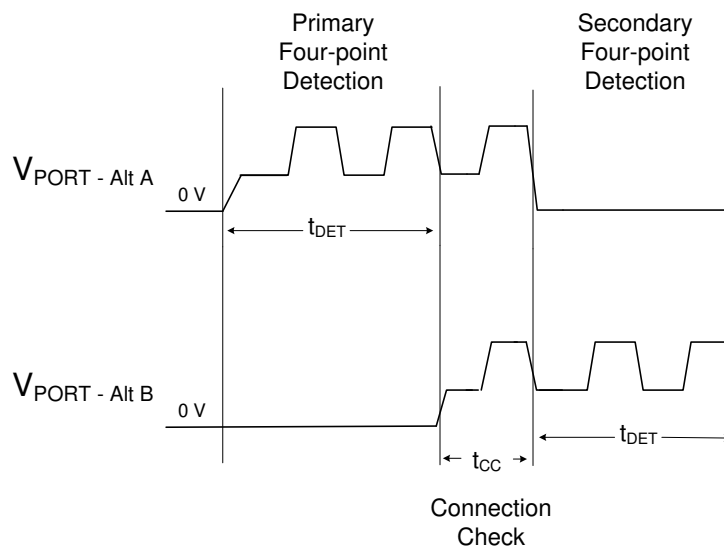
图 8-4. 在单一特征负载条件下 4 线对端口的检测和连接检查波形
