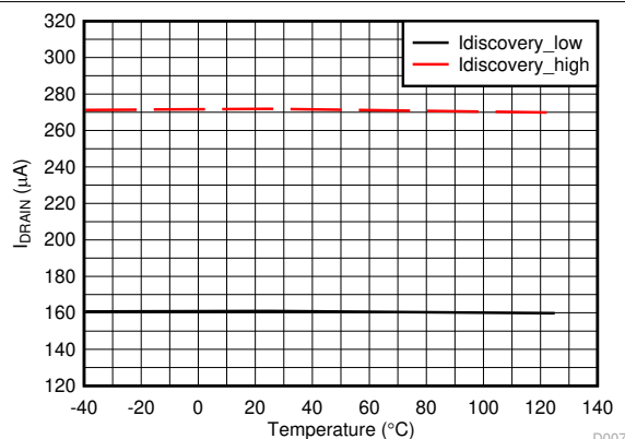
图 6-7. 发现电流与温度间的关系
