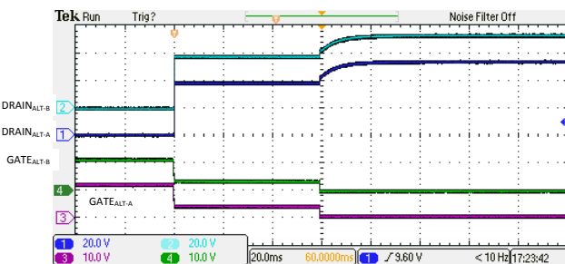
图 9-6. 4 线对 I_{LIM} 折返和关闭
