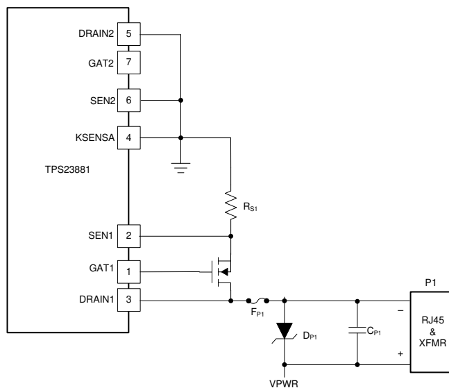
图 9-3. 未使用的 PORT2 的连接
