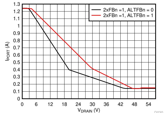
图 6-30. 2x 模式 ( 2\text{xFBn} = 1 ) 电流折返与漏极电压间的关系
