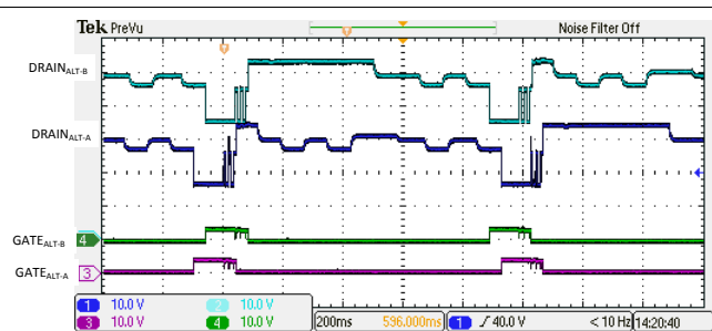
图 9-23. 具有有效双特征 4D 级负载的 4 线对半自动模式发现
