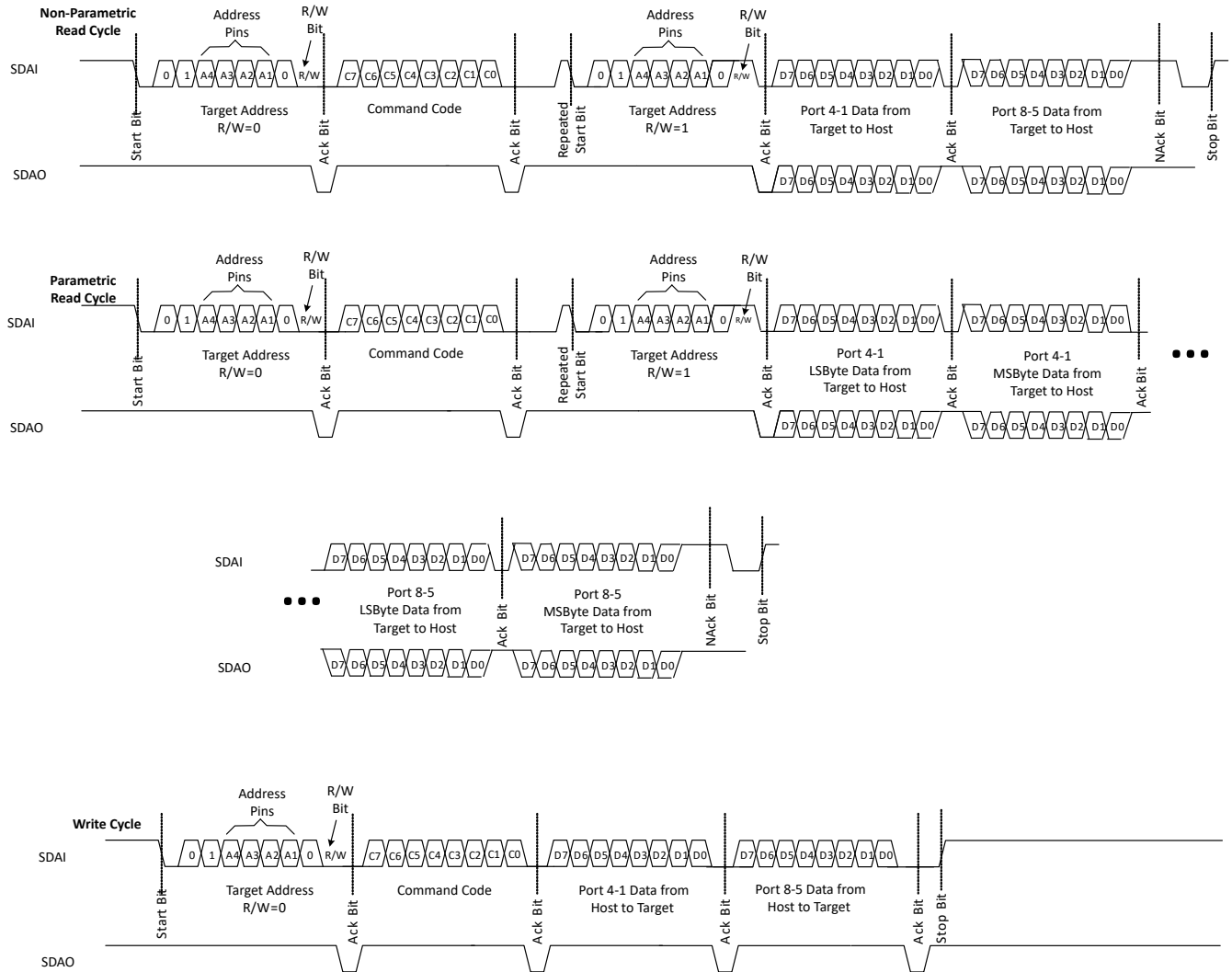
图 8-7. I 2 C 接口读写协议 - 配置 B
