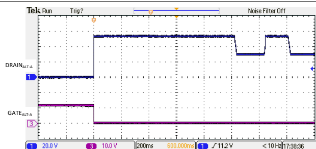
图 9-5. 由于 PCut 故障导致的 2 线对退避
