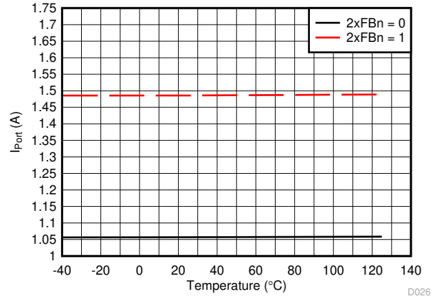
图 6-26. I_{\text{SHORT}} 阈值与温度间的关系
