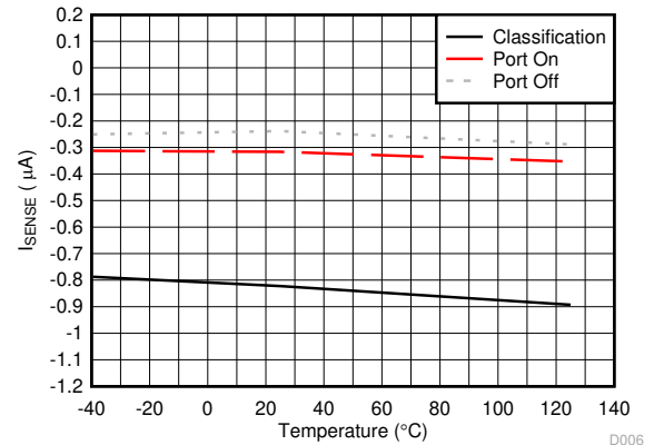
图 6-6. SENSE 引脚偏置电流与温度间的关系
