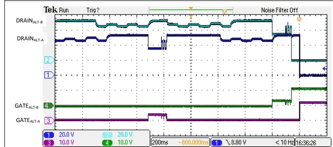
图 9-18. 半自动模式下的 4 线对单一特征发现和开启
