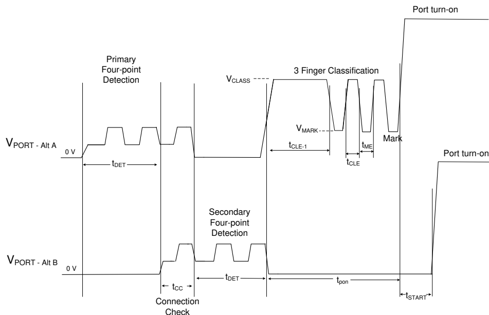
图 7-5. 4 线对单一特征检测、3 事件分级和开启
