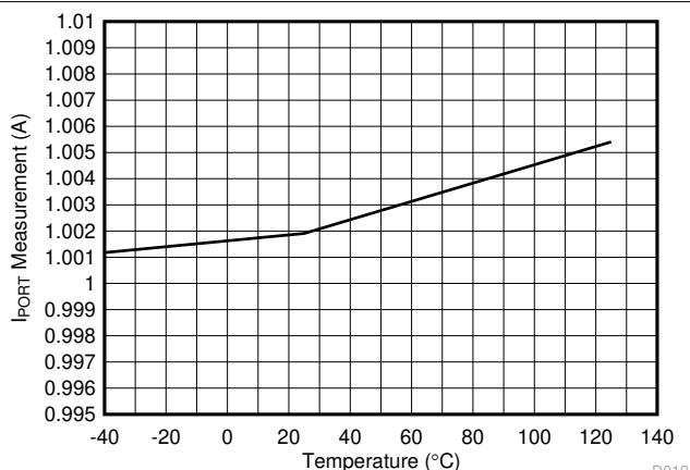
图 6-19. 端口电流 ADC 测量值 (1A) 与温度间的关系
