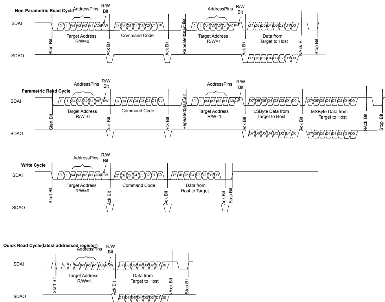
图 8-6. I 2 C 接口读写协议 - 配置 A
