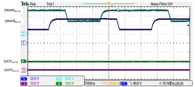
图 9-11. 4 线对开路检测特征
