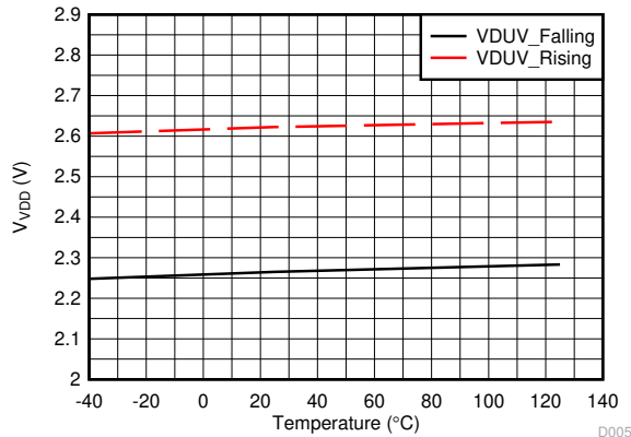
图 6-5. VDUV 阈值与温度间的关系
