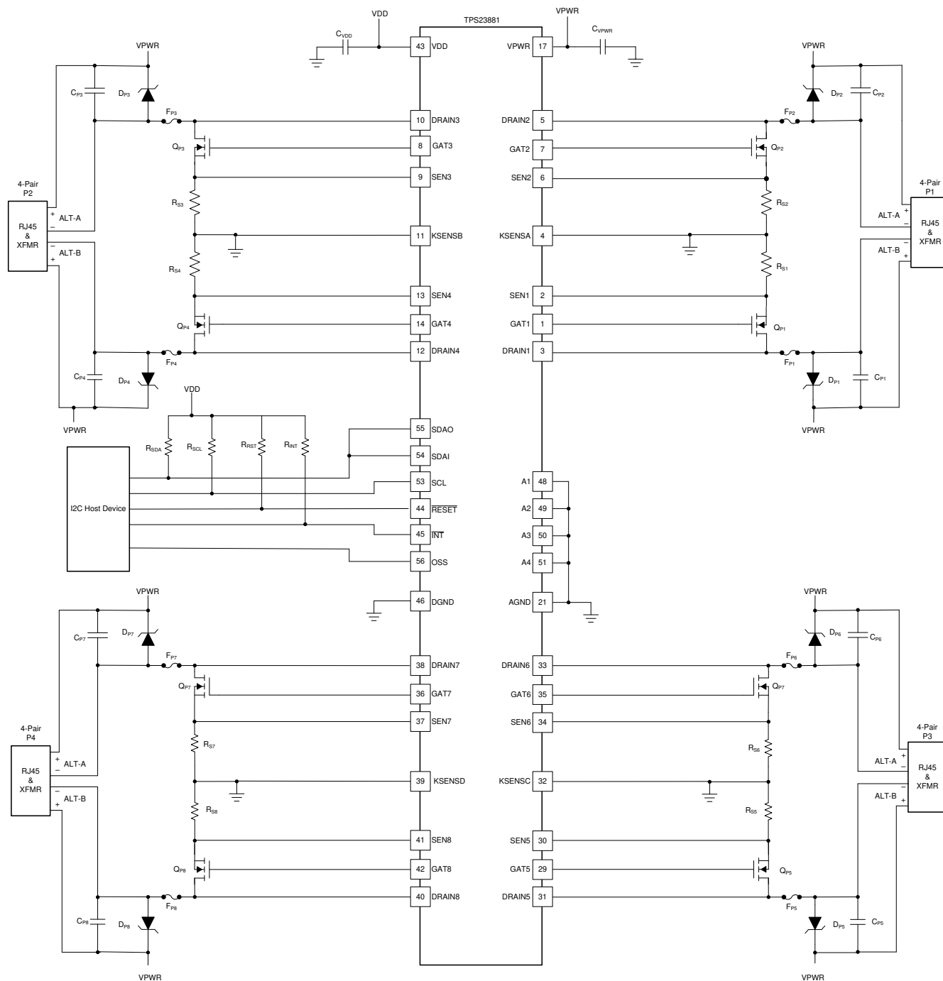
图 9-2. 四 ( 4 线对 ) 端口应用
