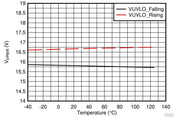
图 6-2. VPWR UVLO 阈值与温度间的关系
