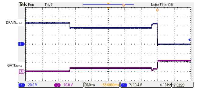
图 9-15. 2 线对 1 级侦测分类和开启
