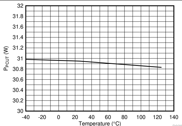
图 6-20. 2 线对 PCut 阈值 (30W) 与温度间的关系
