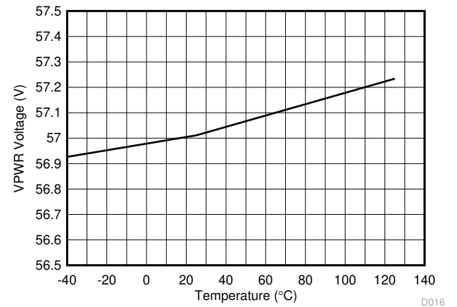
图 6-16. VPWR 电压 ADC 测量值与温度间的关系
