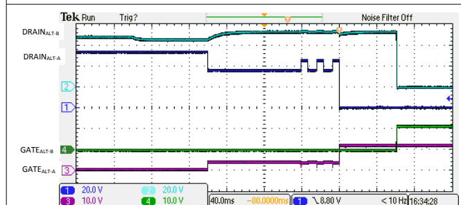
图 9-20. 4 线对单一特征 3 级侦测分级和开启
