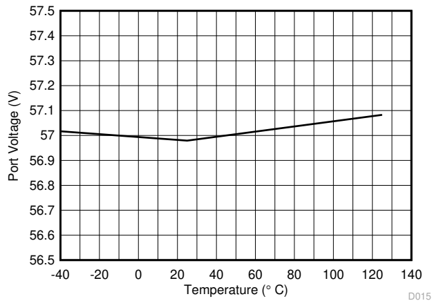
图 6-15. 端口电压 ADC 测量值与温度间的关系
