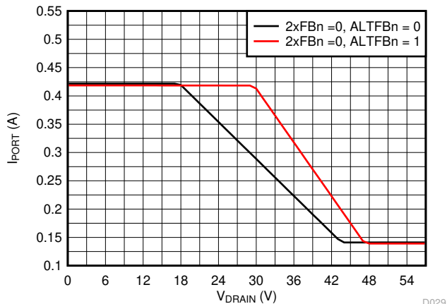
图 6-29. 1x 模式 ( 2\text{xFBn} = 0 ) 电流折返与漏极电压间的关系
