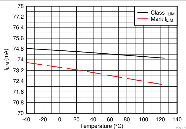
图 6-12. 分级和标记电流限制与温度间的关系
