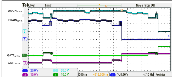
图 9-24. 半自动模式下的 4 线对双特征发现和开启
