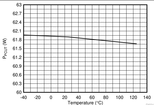
图 6-21. 4 线对 PCut 阈值 (60W) 与温度间的关系
