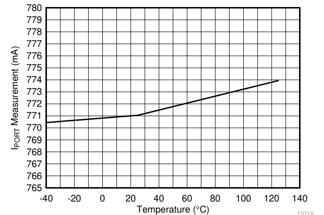
图 6-18. 端口电流 ADC 测量值 (770mA) 与温度间的关系
