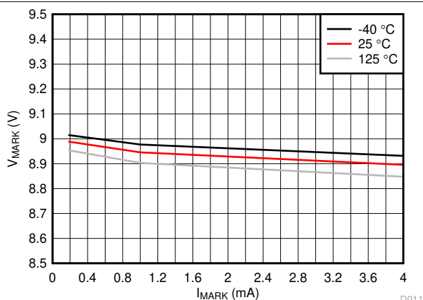
图 6-11. 标记电压与 I_{\text{MARK}} 和温度间的关系
