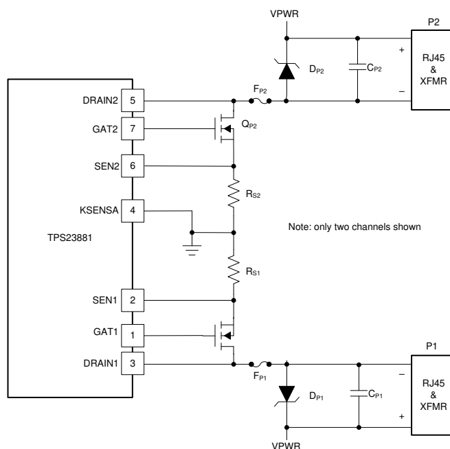
图 9-28. 开尔文电流检测连接
