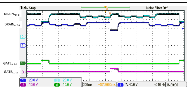
图 9-17. 具有有效单一特征 0-3 级负载的 4 线对半自动模式发现
