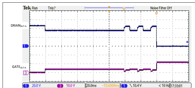
图 9-16. 2 线对 3 级侦测分类和开启
