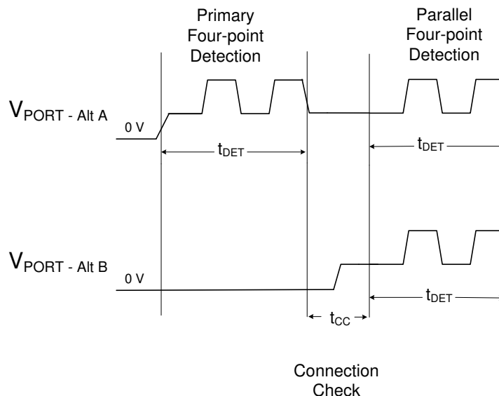
图 8-5. 在双特征负载条件下 4 线对端口的检测和连接检查波形
