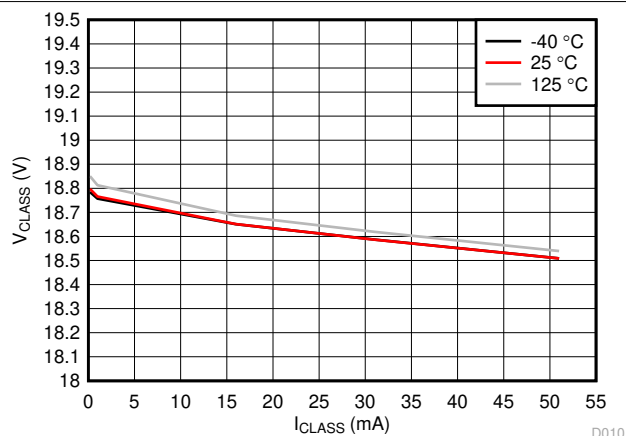
图 6-10. 分级电压与 I_{\text{CLASS}} 和温度间的关系
