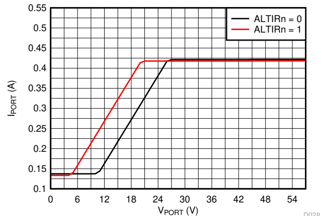
图 6-28. 浪涌电流折返与端口电压间的关系
