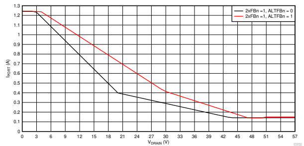
图 8-80. 2x 模式 (2xFBn = 1) 折返曲线， I_{PORT} 与 V_{DRAIN} 间的关系
