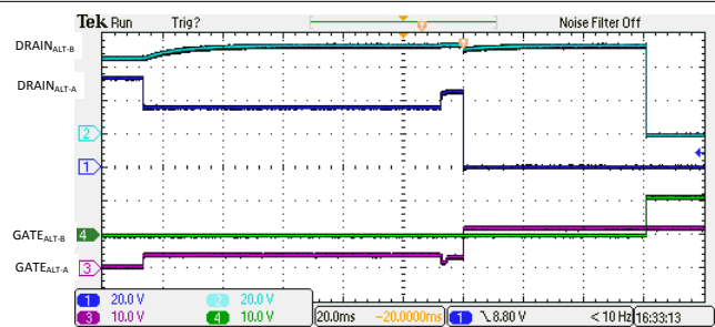
图 9-19. 4 线对单一特征 1 级侦测分级和开启
