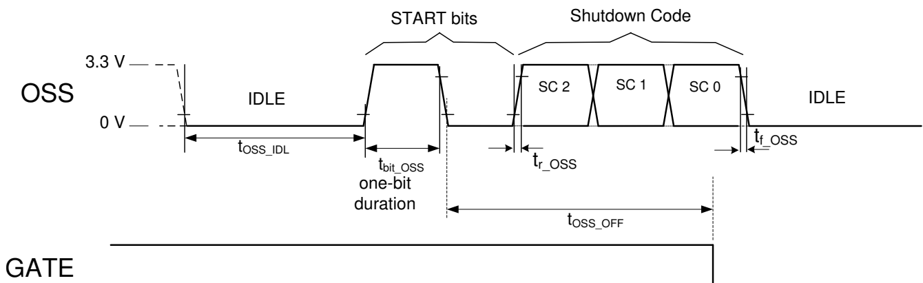
图 8-1. 如果是较低优先级端口，多位优先级端口将关断
