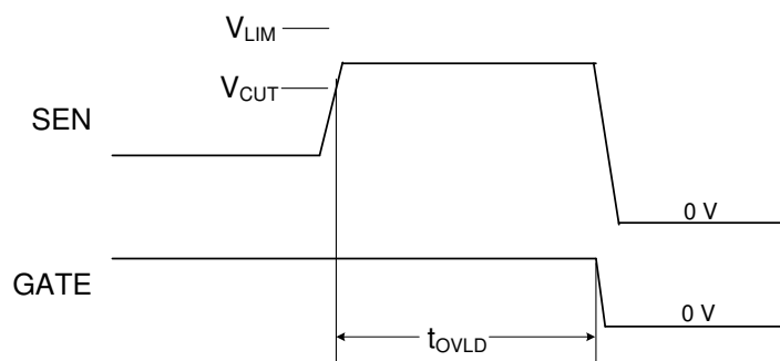
图 7-2. 过流故障时序
