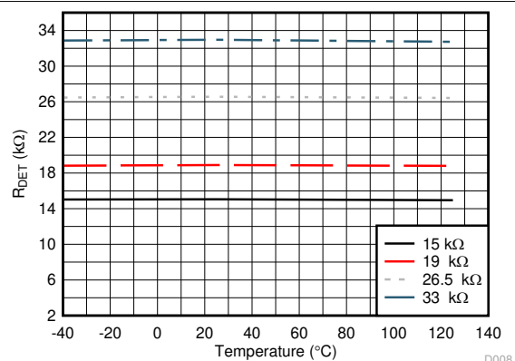
图 6-8. 发现电阻测量值与温度间的关系
