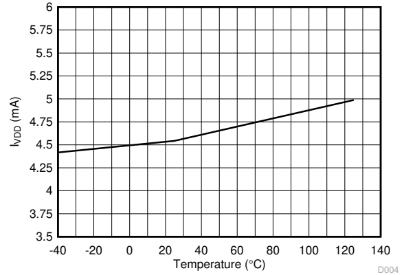
图 6-4. VDD 电流消耗与温度间的关系
