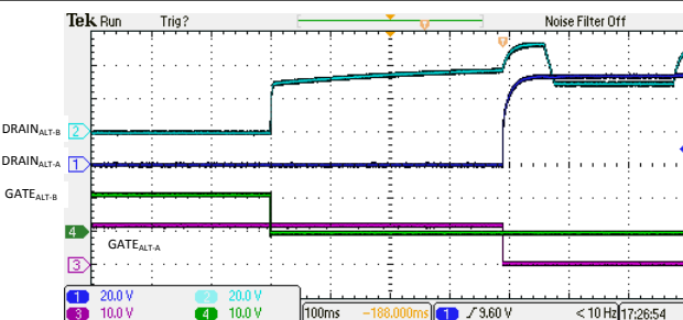
图 9-9. 4 线对单一特征 0-4 级断开
