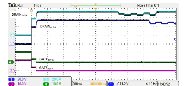
图 9-7. 由于 I_{LIM} 故障导致的 4 线对退避
