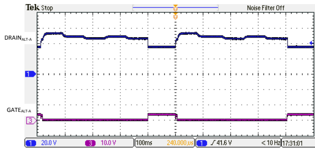
图 9-14. 具有有效 0-3 类负载的 2 线对半自动模式发现
