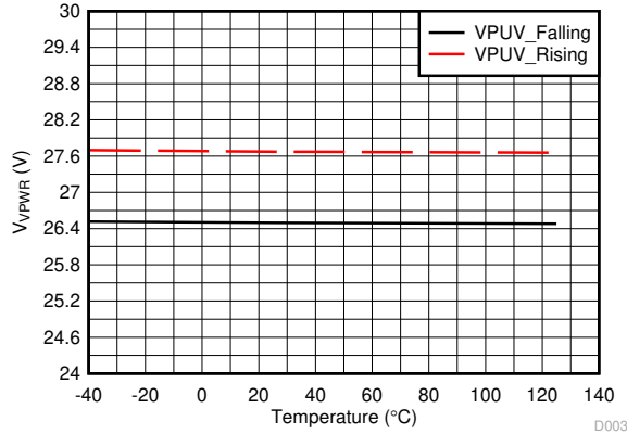
图 6-3. VPUV 阈值与温度间的关系
