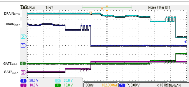
图 9-27. 4 线对双特征 4 级侦测分级和开启
