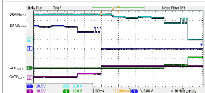
图 9-26. 4 线对双特征 3 级侦测分级和开启
