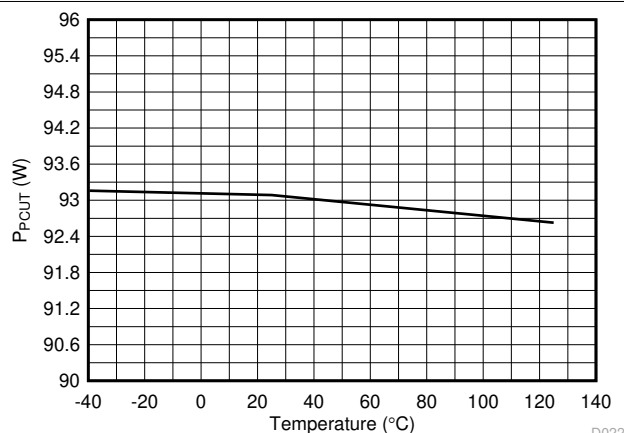
图 6-22. 4 线对 PCut 阈值 (90W) 与温度间的关系
