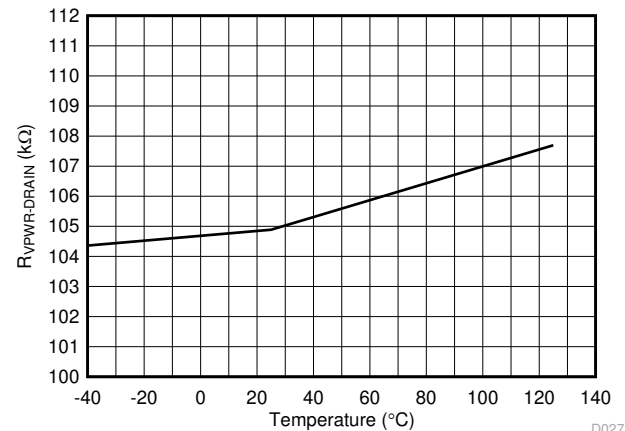
图 6-27. R_{\text{OFF}} (VPWR 至 DRAIN) 与温度间的关系
