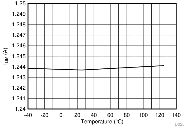
图 6-25. 2x 模式 (2xFBn = 1) 电流限制与温度间的关系
