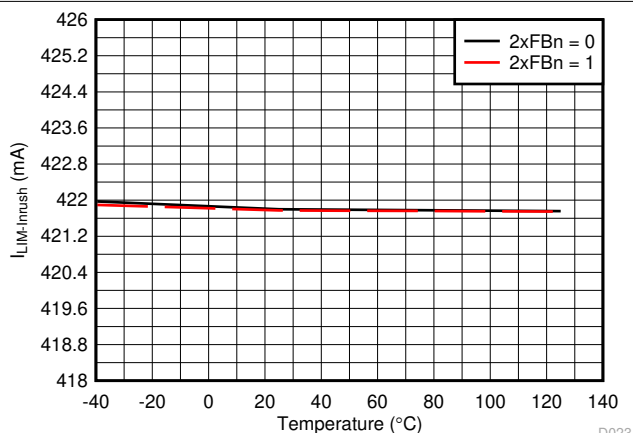
图 6-23. 浪涌电流限制与温度间的关系
