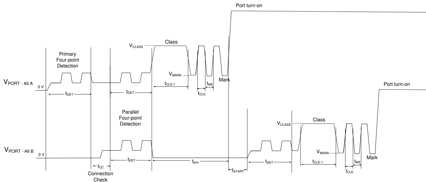
图 7-7. 4 线对双特征检测、3 事件分级和开启
