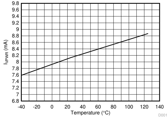
图 6-1. VPWR 电流消耗与温度间的关系
