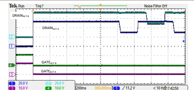
图 9-8. 由于 4PPCut 故障导致的 4 线对退避
