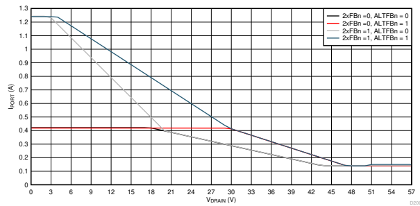
图 8-3. 端口已开启时折返 : I_{LIM} 与 V_{drain} 间的关系
