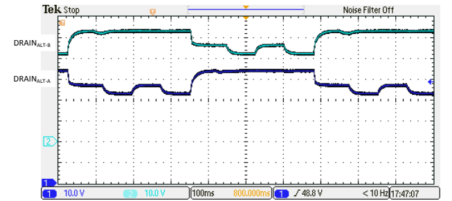
图 9-13. 4 线对高电阻 (36k \Omega ) 检测特征
