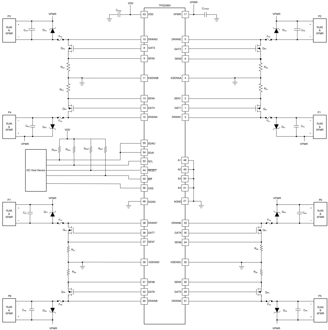
图 9-1. 八 (2 线对) 端口应用
