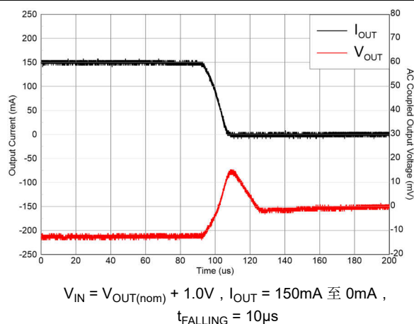
图 5-12. 负载瞬态
